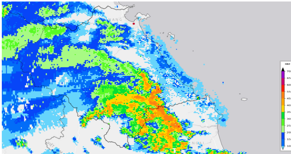
Hình 1: Ảnh ra đa Tam Kỳ lúc 18h45 ngày 11/8/2025
