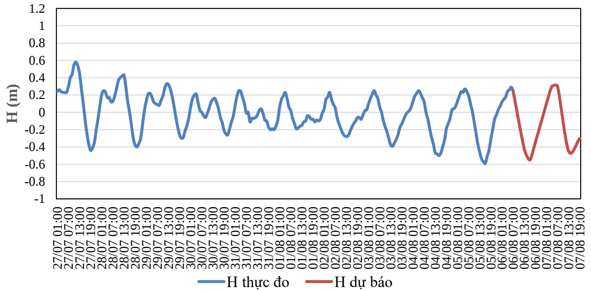
QUÁ TRÌNH MỨC NƯỚC THỰC ĐO VÀ DỰ BÁO TRẠM HỘI AN (Từ 01h/27/7 đến 07h/7/8/2025)
