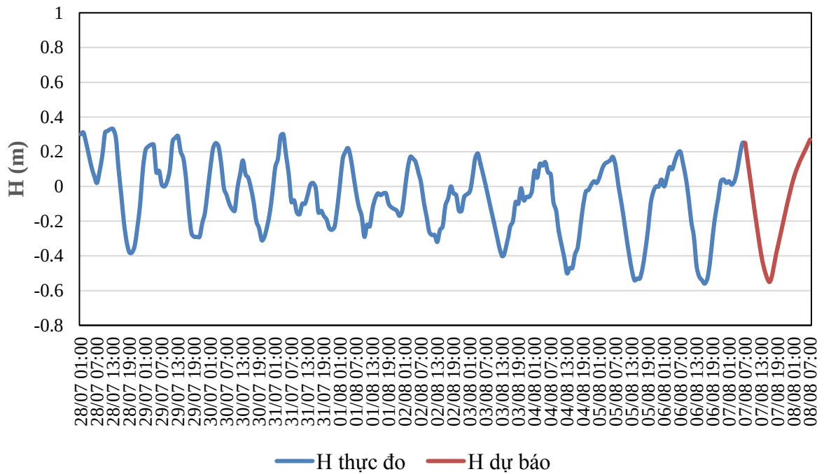
QUÁ TRÌNH MỨC NƯỚC THỰC ĐO VÀ DỰ BÁO TRẠM CẨM LỆ (Từ 01h/28/7 đến 07h/8/8/2025)
