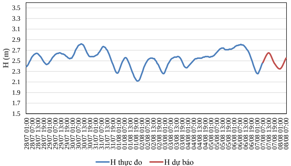
QUÁ TRÌNH MỨC NƯỚC THỰC ĐO VÀ DỰ BÁO TRẠM ÁI NGHĨA (Từ 01h/28/7 đến 07h/8/8/2025)
