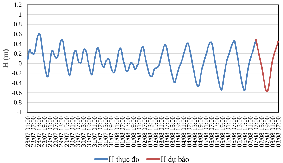
QUÁ TRÌNH MỨC NƯỚC THỰC ĐO VÀ DỰ BÁO TRẠM TAM KỲ (Từ 01h/28/7 đến 07h/8/8/2025)
