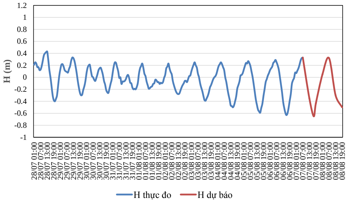
QUÁ TRÌNH MỨC NƯỚC THỰC ĐO VÀ DỰ BÁO TRẠM HỘI AN (Từ 01h/28/7 đến 07h/8/8/2025)
