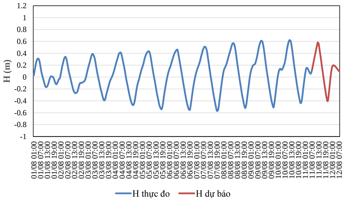
QUÁ TRÌNH MỨC NƯỚC THỰC ĐO VÀ DỰ BÁO TRẠM TAM KỲ (Từ 01h/1/8 đến 07h/12/8/2025)
