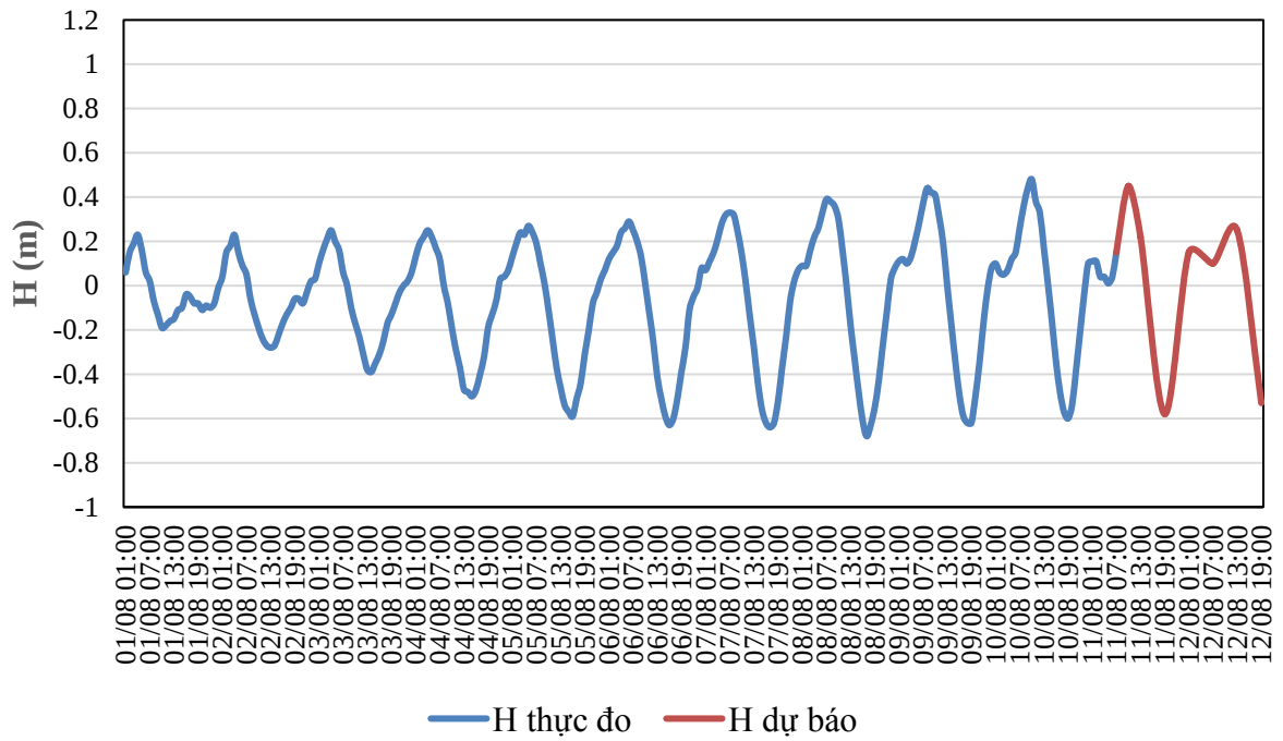
QUÁ TRÌNH MỨC NƯỚC THỰC ĐO VÀ DỰ BÁO TRẠM HỘI AN (Từ 01h/1/8 đến 07h/12/8/2025)
