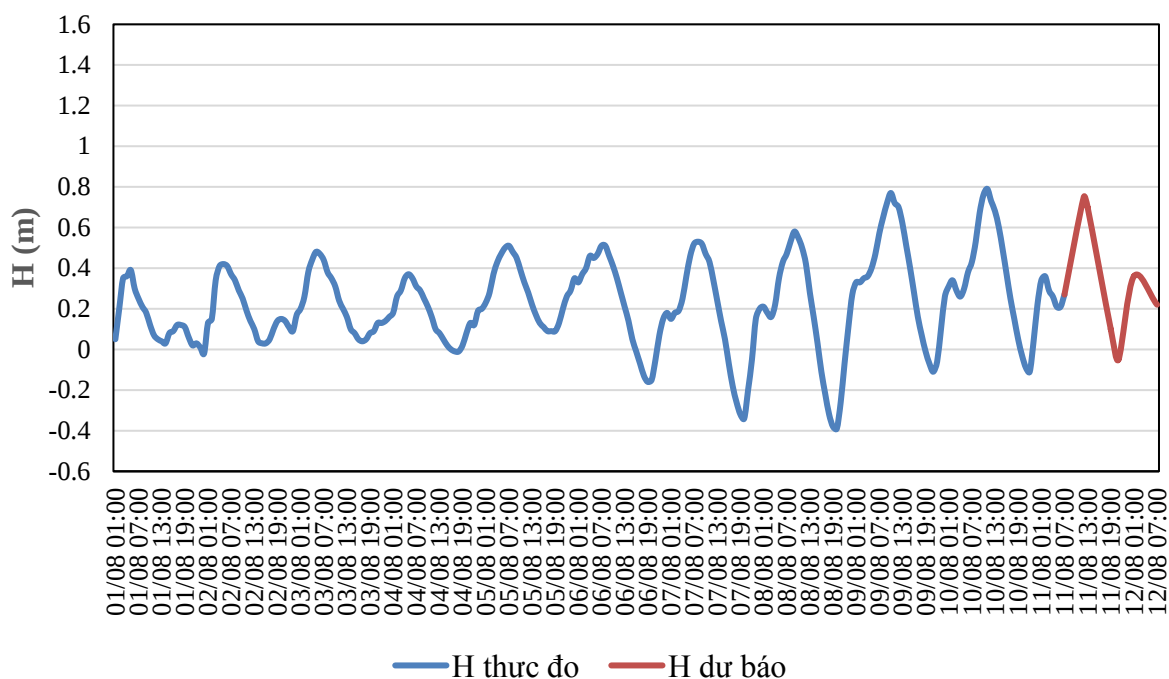
QUÁ TRÌNH MỨC NƯỚC THỰC ĐO VÀ DỰ BÁO TRẠM GIAO THỦY (Từ 01h/1/8 đến 07h/12/8/2025)
