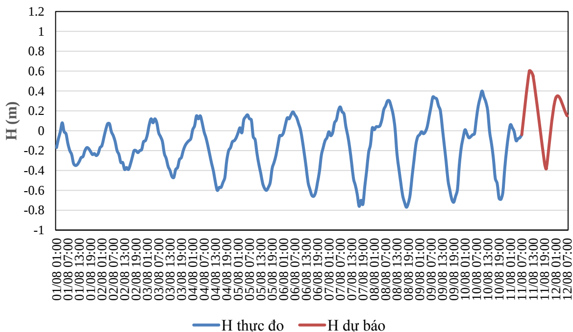
QUÁ TRÌNH MỨC NƯỚC THỰC ĐO VÀ DỰ BÁO TRẠM CÂU LÂU (Từ 01h/1/8 đến 07h/12/8/2025)
