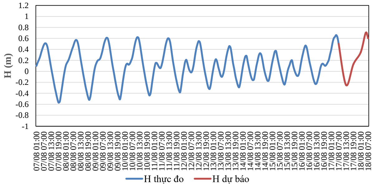
QUÁ TRÌNH MỨC NƯỚC THỰC ĐO VÀ DỰ BÁO TRẠM TAM KỲ (Từ 01h/7/8 đến 07h/18/8/2025)
