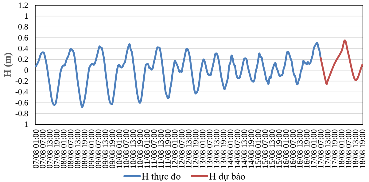
QUÁ TRÌNH MỨC NƯỚC THỰC ĐO VÀ DỰ BÁO TRẠM HỘI AN (Từ 01h/7/8 đến 07h/18/8/2025)
