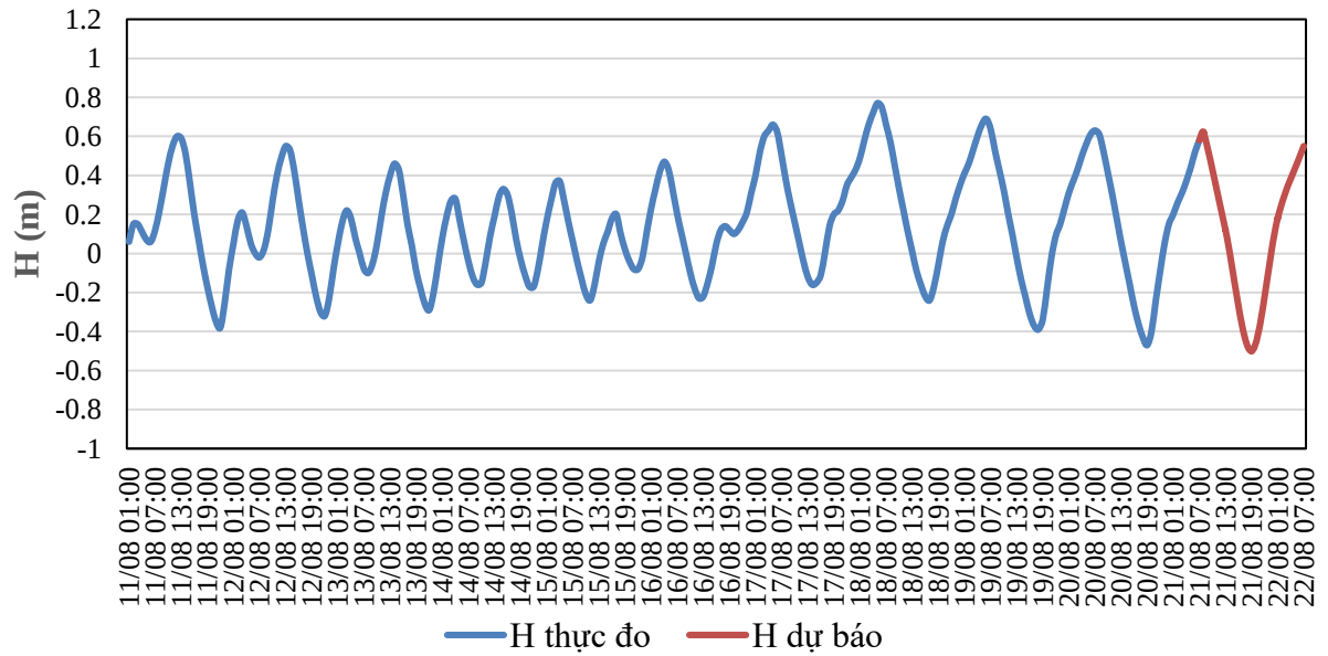
QUÁ TRÌNH MỨC NƯỚC THỰC ĐO VÀ DỰ BÁO TRẠM TAM KỲ (Từ 01h/11/8 đến 07h/22/8/2025)
