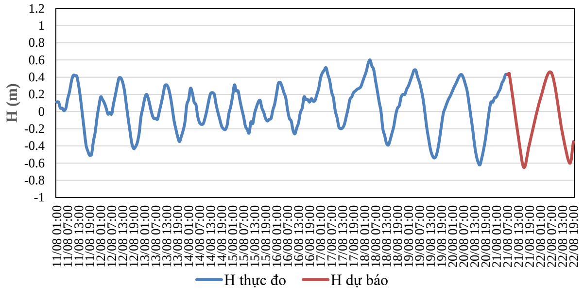
QUÁ TRÌNH MỨC NƯỚC THỰC ĐO VÀ DỰ BÁO TRẠM HỘI AN (Từ 01h/11/8 đến 07h/22/8/2025)
