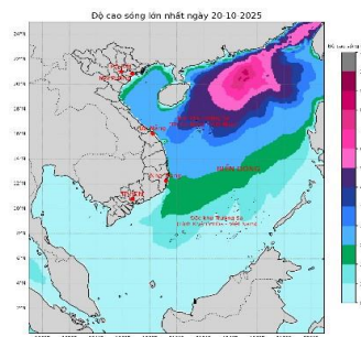
Hình 1: Bản đồ dự báo gió mạnh, sóng lớn trong 24h tới
