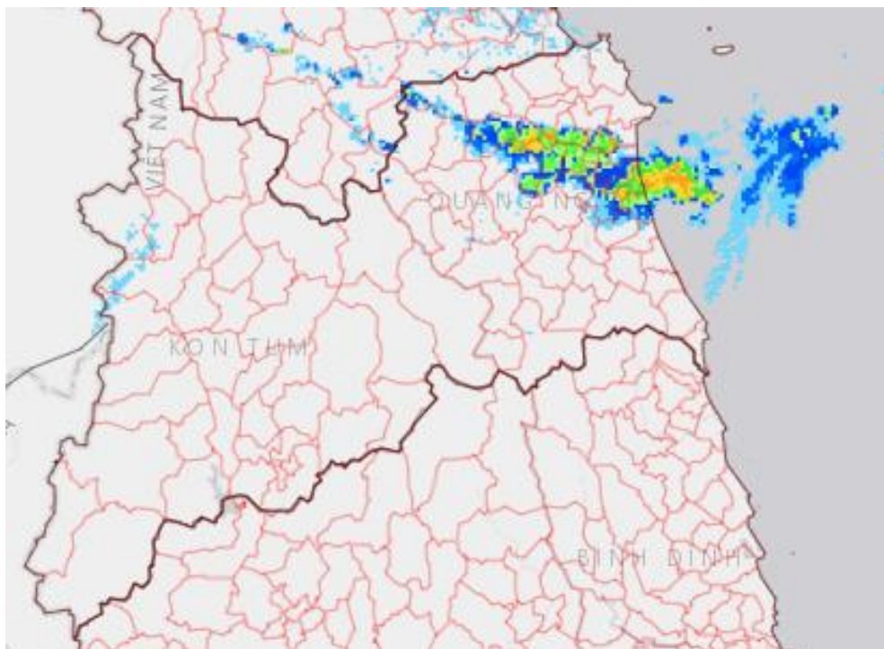
Hình ra đa lúc 09h50 ngày 30/10/2025
