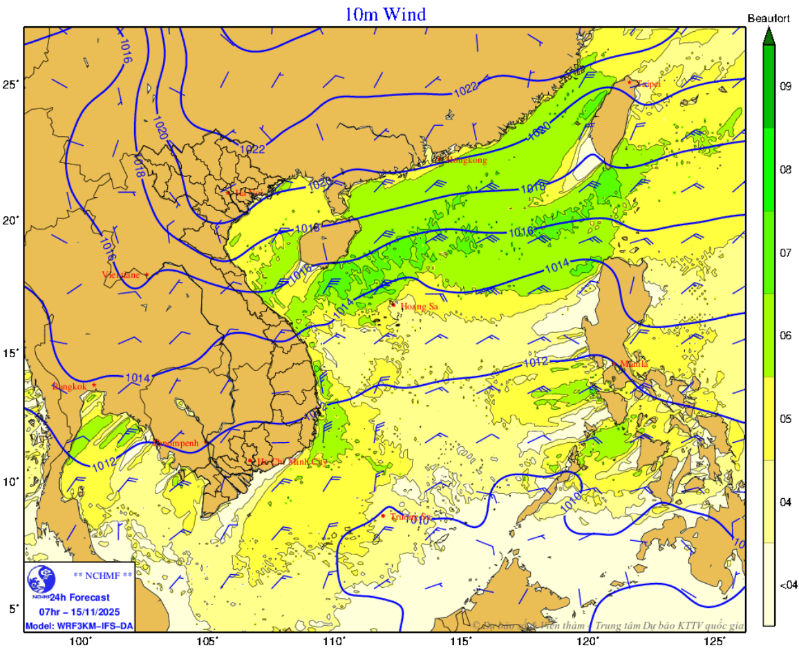
Hình. Bản đồ dự báo gió mạnh lúc 07h ngày 15/11
