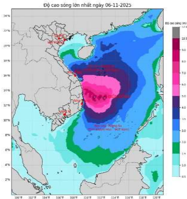
Hình 1. Bản đồ dự báo độ cao sóng
