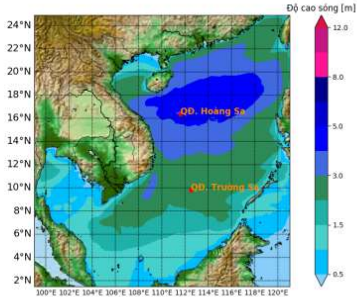
Hình 1. Bản đồ dự báo độ cao sóng
