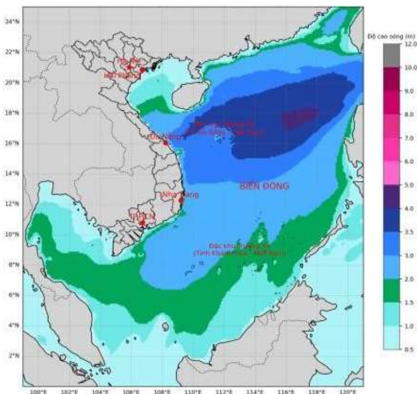
Hình 1. Bản đồ dự báo độ cao sóng
