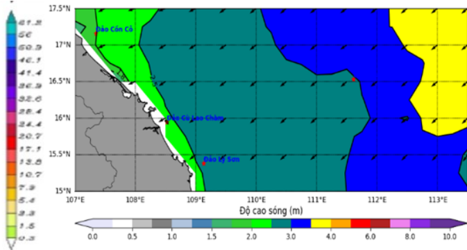
Hình 1: Bản đồ dự báo gió mạnh 24 giờ tới Hình 2: Bản đồ dự báo sóng lớn 24 giờ tới
