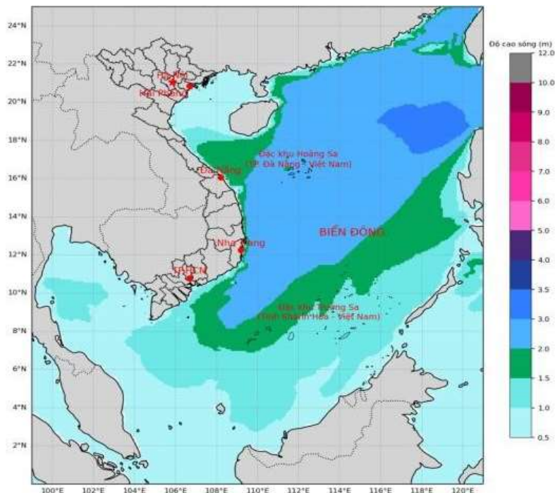
Hình 1. Bản đồ dự báo độ cao sóng
