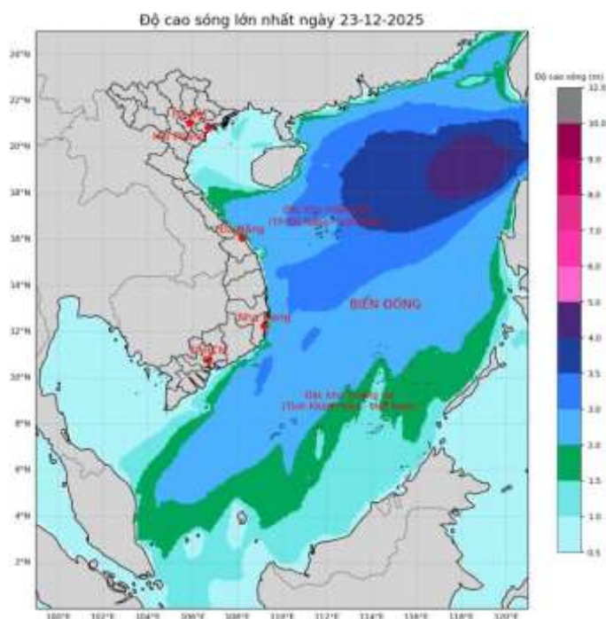
Hình 1. Bản đồ dự báo độ cao sóng
