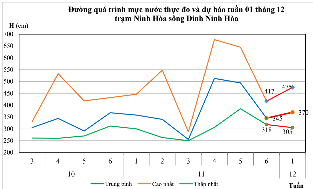
Hình 1: Quá trình mực nước thực đo và dự báo trạm Ninh Hòa từ ngày 01/12 đến ngày 05/12
