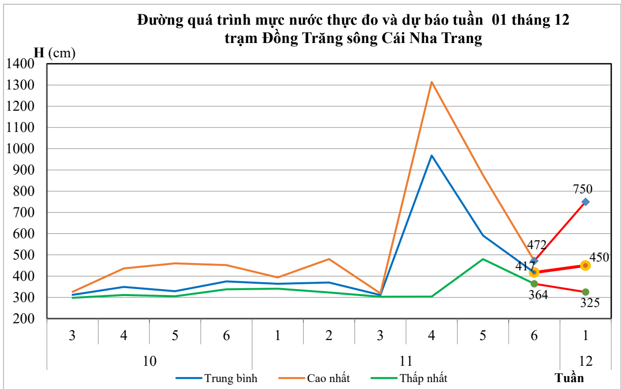
Hình 2: Quá trình mực nước thực đo và dự báo trạm Đồng Trăng từ ngày 01/12 đến ngày 05/12
