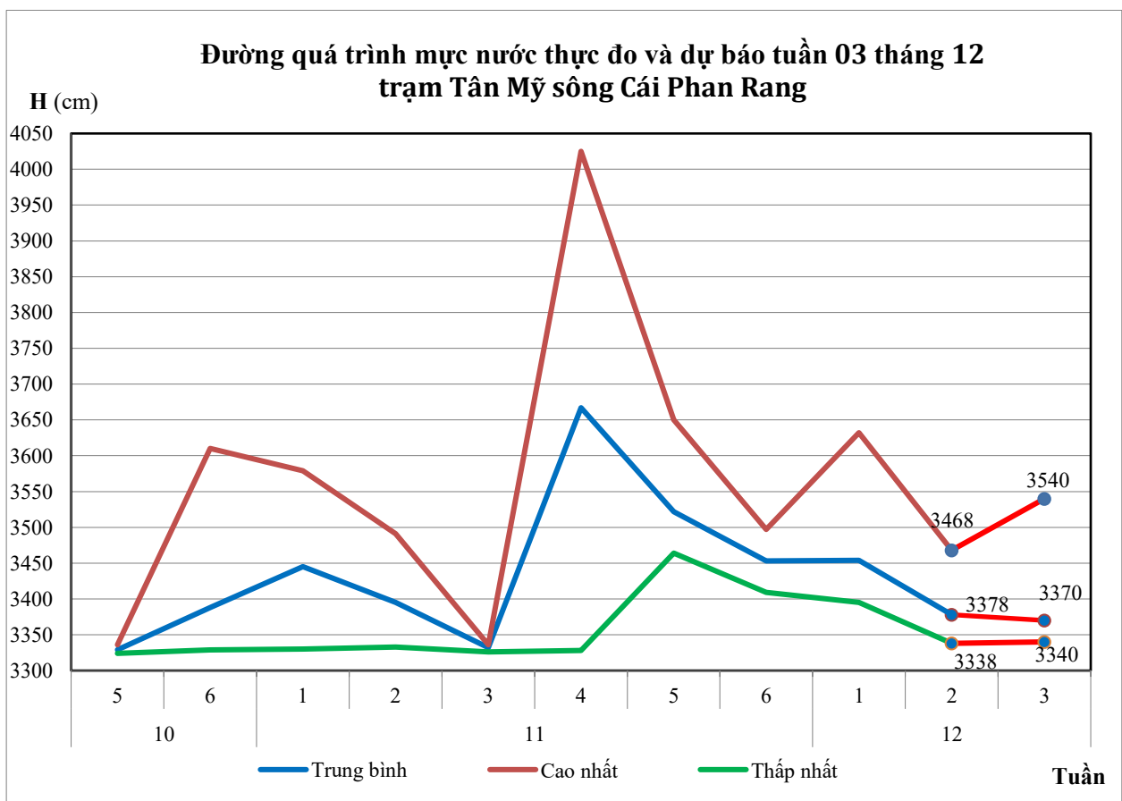
Hình 3: Quá trình mực nước thực đo và dự báo trạm Tân Mỹ từ ngày 11/12 đến ngày 15/12
