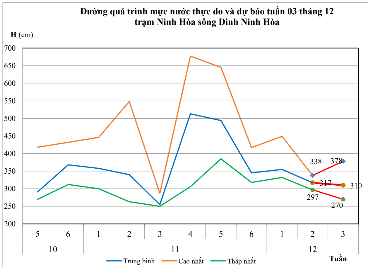
Hình 1: Quá trình mực nước thực đo và dự báo trạm Ninh Hòa từ ngày 11/12 đến ngày 15/12
