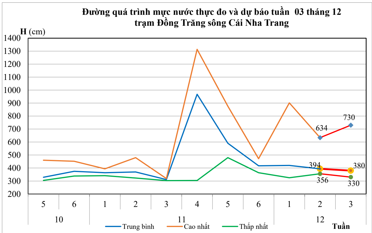
Hình 2: Quá trình mực nước thực đo và dự báo trạm Đồng Trăng từ ngày 11/12 đến ngày 15/12
