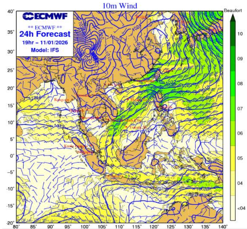
Hình 1. Sản phẩm dự báo gió lúc 19h ngày 11/01/2026
