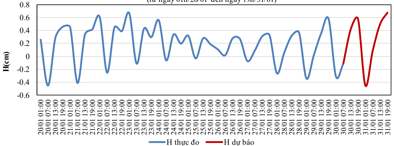
QUÁ TRÌNH MỨC NƯỚC THỰC ĐO VÀ DỰ BÁO TRẠM THỦY VĂN HỘI AN (từ ngày 01h/20/01 đến ngày 19h/31/01)
