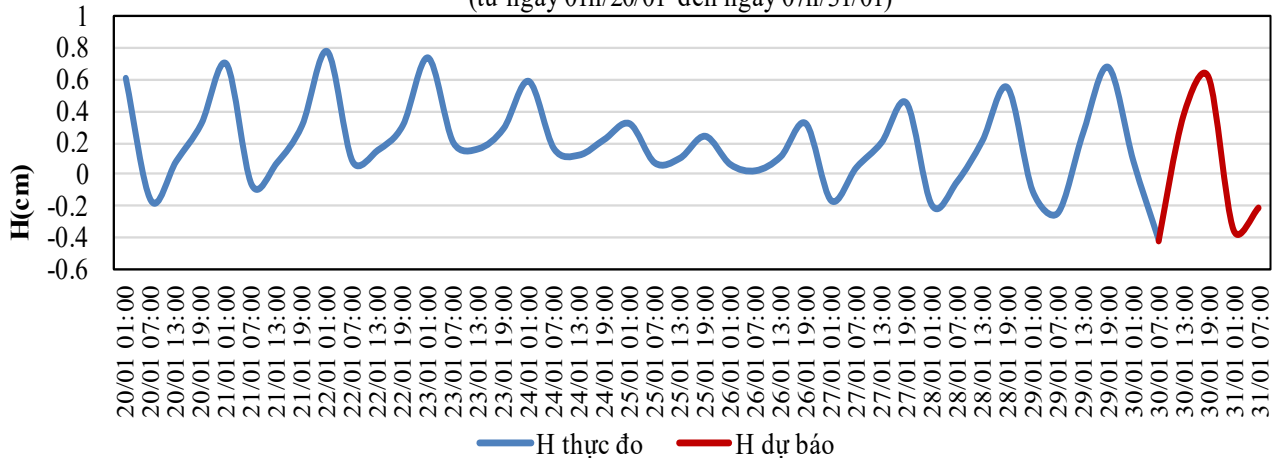
QUÁ TRÌNH MỨC NƯỚC THỰC ĐO VÀ DỰ BÁO TRẠM THỦY VĂN TAM KỶ (từ ngày 01h/20/01 đến ngày 07h/31/01)
