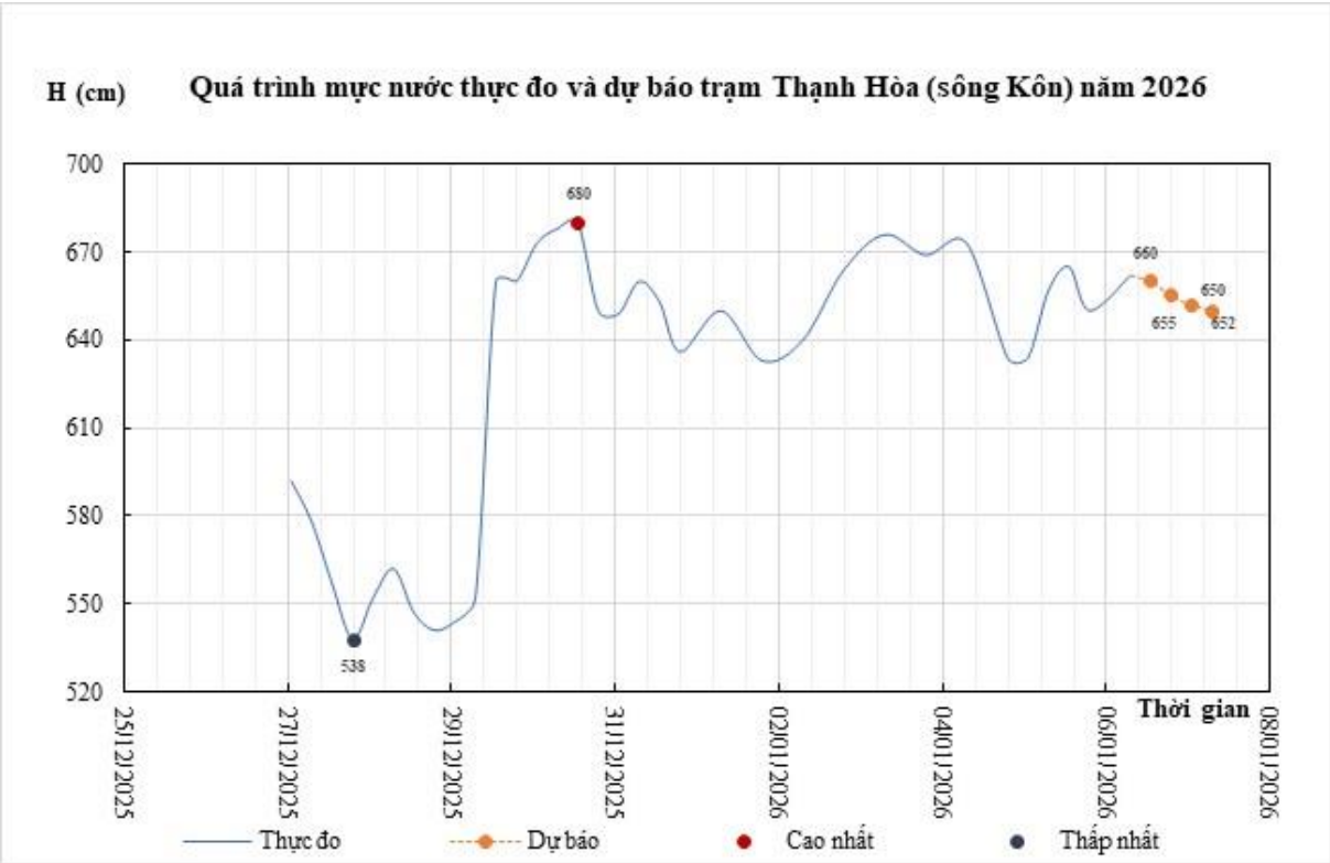
Hình 8: Quá trình mực nước thực đo và dự báo trạm thủy văn Thạnh Hòa
