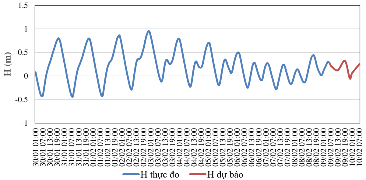
QUÁ TRÌNH MỨC NƯỚC THỰC ĐO VÀ DỰ BÁO TRẠM TAM KỶ (Từ 01h/30/1 đến 07h/10/2/2026)
