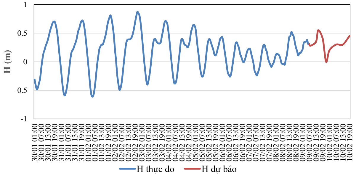
QUÁ TRÌNH MỨC NƯỚC THỰC ĐO VÀ DỰ BÁO TRẠM HỘI AN (Từ 01h/30/1 đến 07h/10/2/2026)
