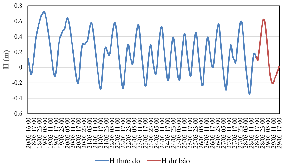
QUÁ TRÌNH MỨC NƯỚC THỰC ĐO VÀ DỰ BÁO TRẠM TAM KỲ (Từ 01h/14/3 đến 07h/25/3/2026)
