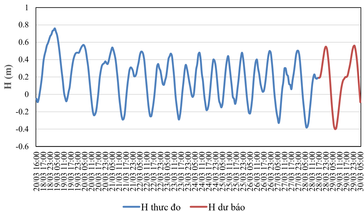
QUÁ TRÌNH MỨC NƯỚC THỰC ĐO VÀ DỰ BÁO TRẠM HỘI AN (Từ 01h/14/3 đến 07h/25/3/2026)
