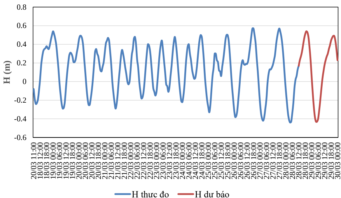
QUÁ TRÌNH MỨC NƯỚC THỰC ĐO VÀ DỰ BÁO TRẠM HỘI AN (Từ 01h/16/3 đến 07h/27/3/2026)
