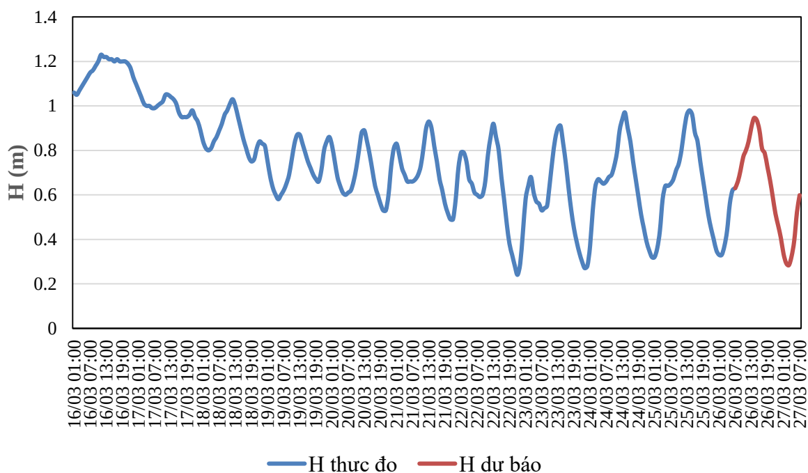
QUÁ TRÌNH MỨC NƯỚC THỰC ĐO VÀ DỰ BÁO TRẠM GIAO THỦY (Từ 01h/16/3 đến 07h/27/3/2026)
