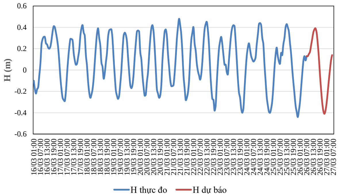
QUÁ TRÌNH MỰC NƯỚC THỰC ĐO VÀ DỰ BÁO TRẠM CẨM LỆ (Từ 01h/16/3 đến 07h/27/3/2026)
