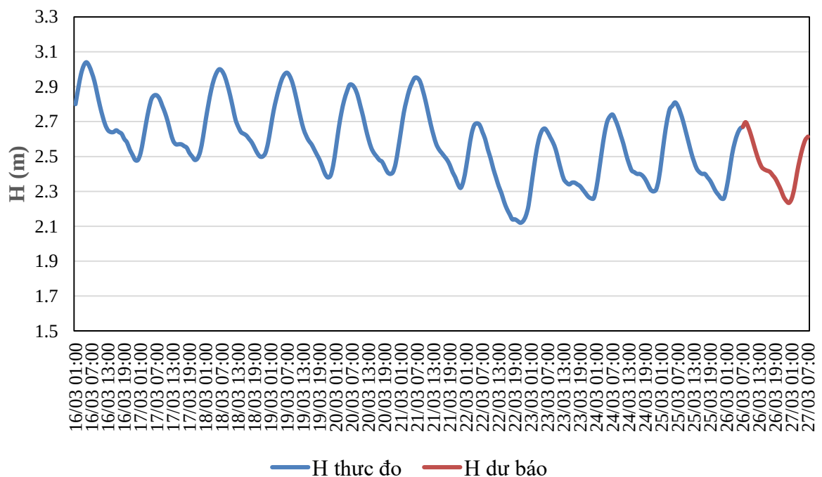
QUÁ TRÌNH MỰC NƯỚC THỰC ĐO VÀ DỰ BÁO TRẠM ÁI NGHĨA (Từ 01h/16/3 đến 07h/27/3/2026)
