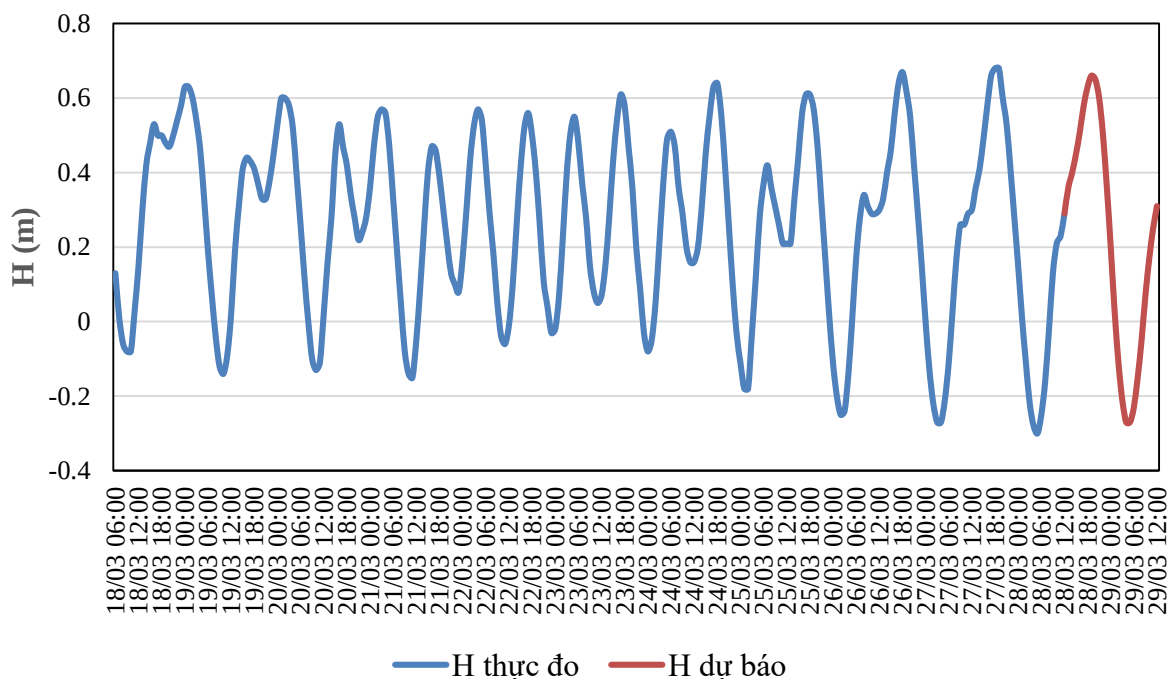
QUÁ TRÌNH MỨC NƯỚC THỰC ĐO VÀ DỰ BÁO TRẠM CÂU LÂU (Từ 01h/16/3 đến 07h/27/3/2026)
