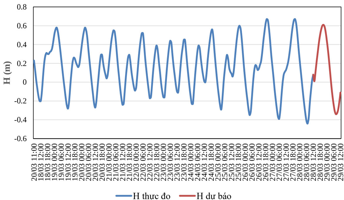
QUÁ TRÌNH MỨC NƯỚC THỰC ĐO VÀ DỰ BÁO TRẠM TAM KỲ (Từ 01h/16/3 đến 07h/27/3/2026)
