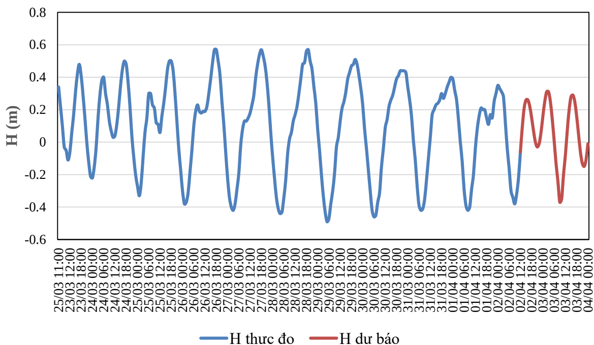
QUÁ TRÌNH MỨC NƯỚC THỰC ĐO VÀ DỰ BÁO TRẠM HỘI AN (Từ 01h/21/3 đến 07h/1/4/2026)
