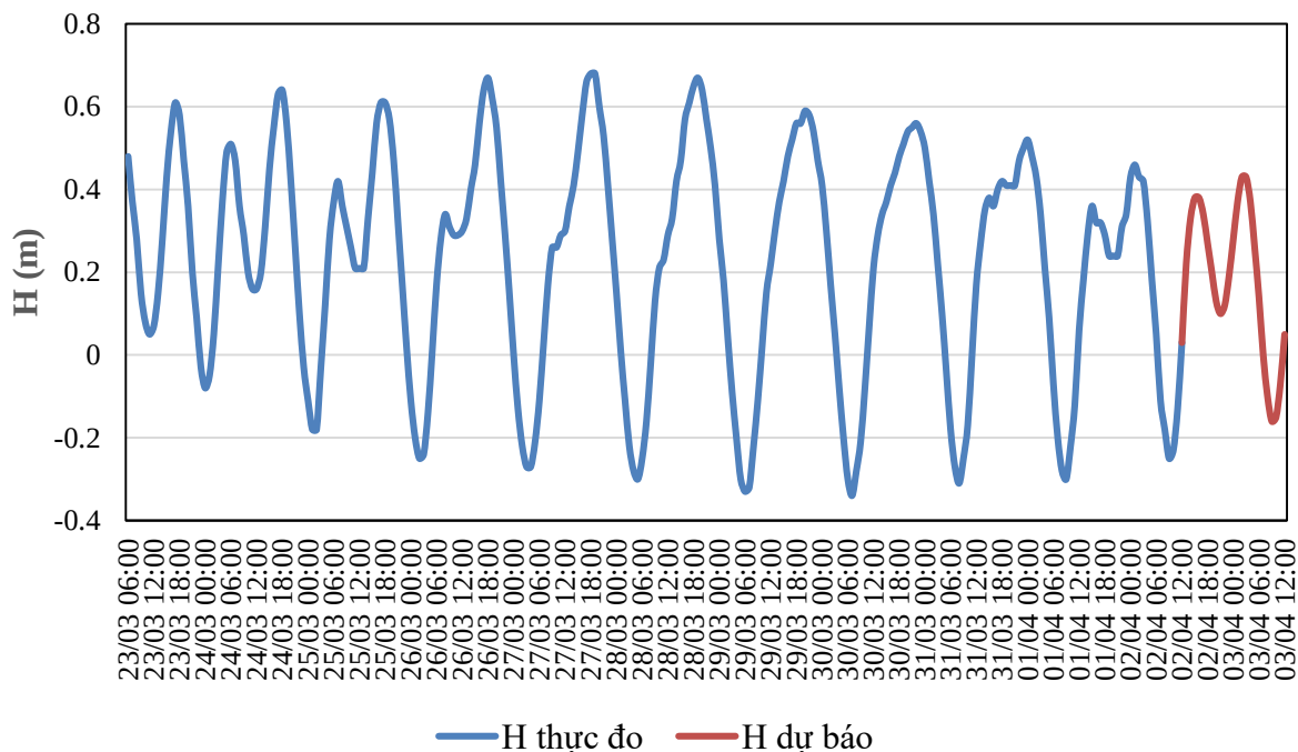
QUÁ TRÌNH MỨC NƯỚC THỰC ĐO VÀ DỰ BÁO TRẠM CÂU LÂU (Từ 01h/21/3 đến 07h/1/4/2026)
