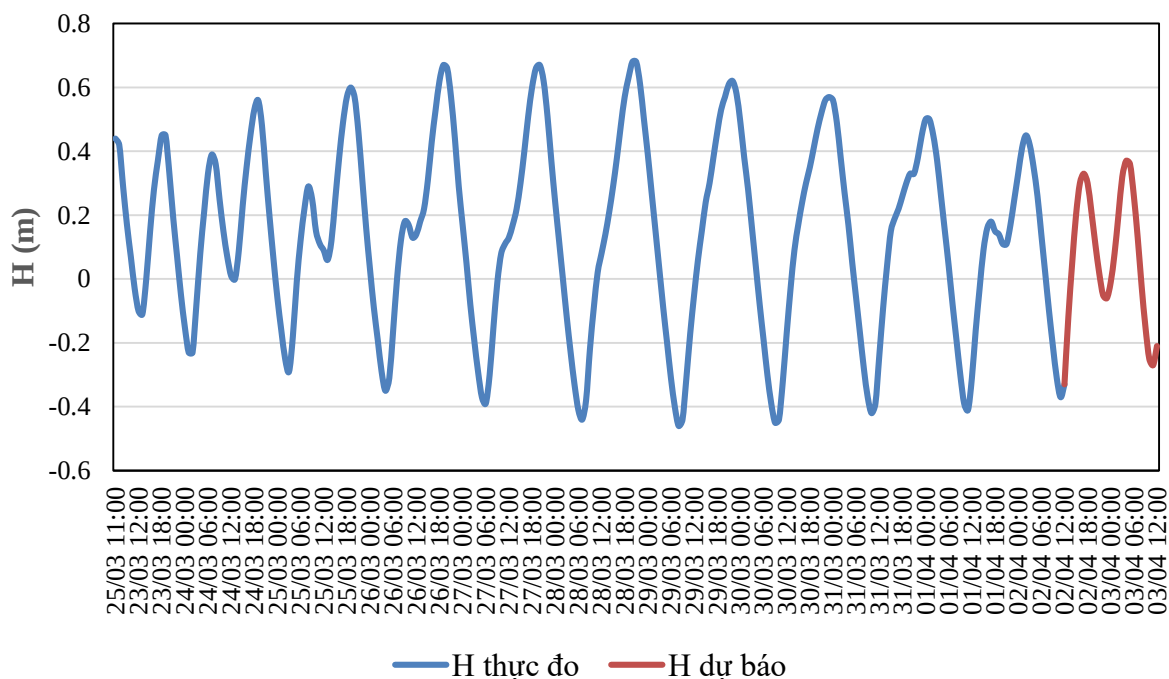
QUÁ TRÌNH MỨC NƯỚC THỰC ĐO VÀ DỰ BÁO TRẠM TAM KỲ (Từ 01h/21/3 đến 07h/1/4/2026)
