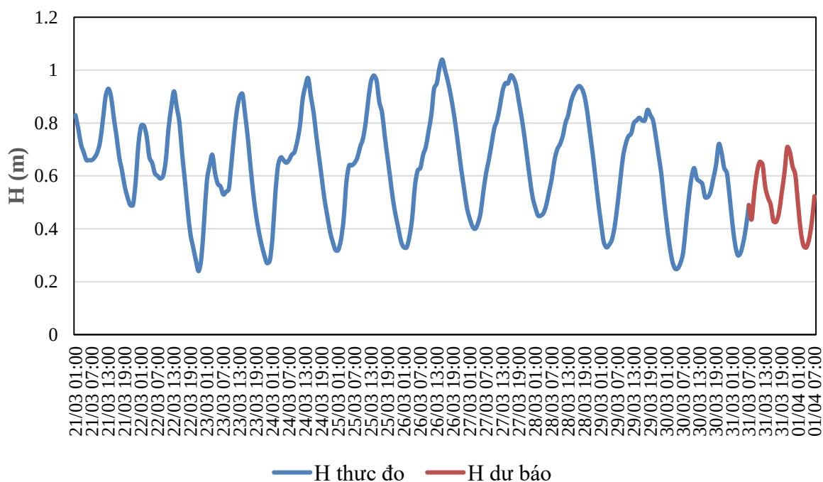
QUÁ TRÌNH MỨC NƯỚC THỰC ĐO VÀ DỰ BÁO TRẠM GIAO THỦY (Từ 01h/21/3 đến 07h/1/4/2026)
