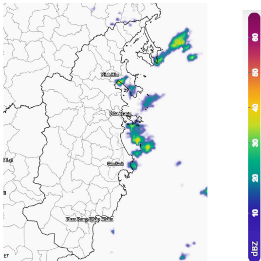
Hình 1: Ảnh radar tại khu vực tỉnh Khánh Hòa
