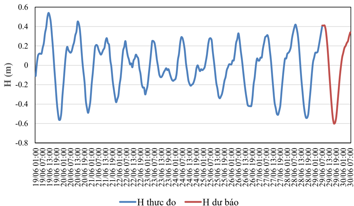
QUÁ TRÌNH MỨC NƯỚC THỰC ĐO VÀ DỰ BÁO TRẠM CÂU LÂU (Từ 01h/19/6 đến 07h/30/6/2026)
