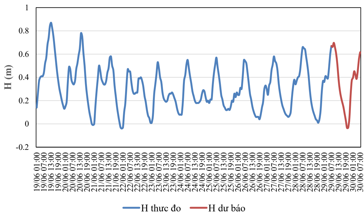
QUÁ TRÌNH MỨC NƯỚC THỰC ĐO VÀ DỰ BÁO TRẠM GIAO THỦY (Từ 01h/19/6 đến 07h/30/6/2026)
