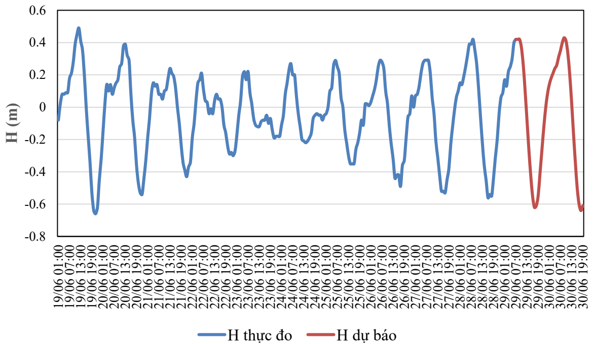
QUÁ TRÌNH MỨC NƯỚC THỰC ĐO VÀ DỰ BÁO TRẠM HỘI AN (Từ 01h/19/6 đến 07h/30/6/2026)
