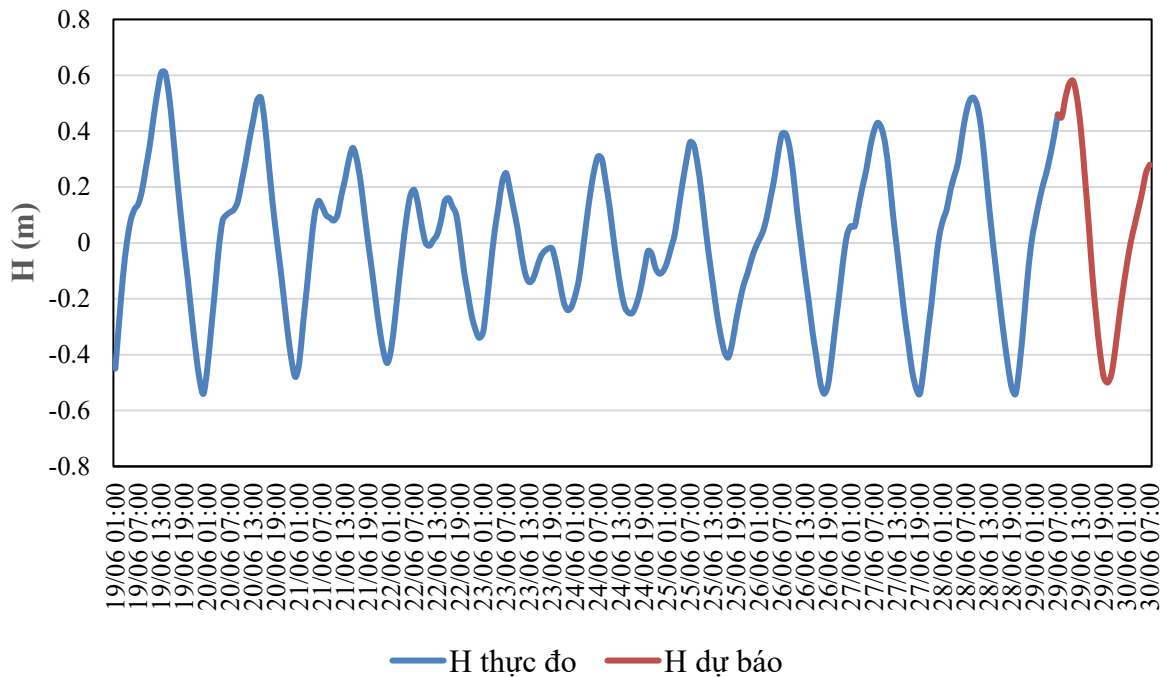
QUÁ TRÌNH MỨC NƯỚC THỰC ĐO VÀ DỰ BÁO TRẠM TAM KỲ (Từ 01h/19/6 đến 07h/30/6/2026)
