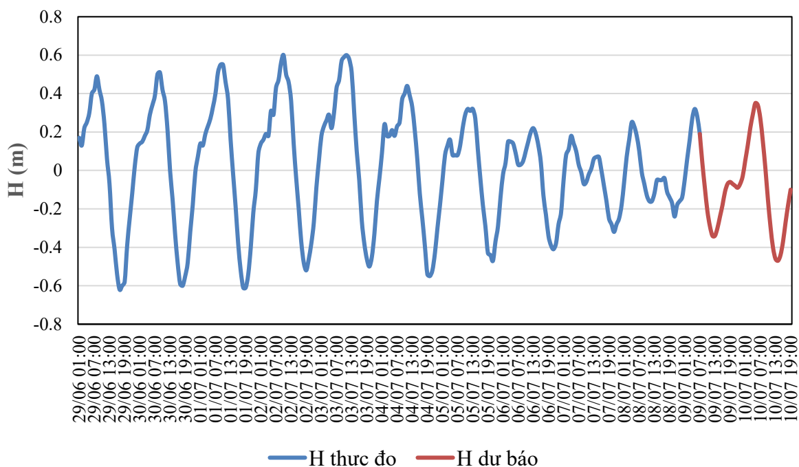
QUÁ TRÌNH MỨC NƯỚC THỰC ĐO VÀ DỰ BÁO TRẠM HỘI AN (Từ 01h/29/6 đến 07h/10/7/2026)
