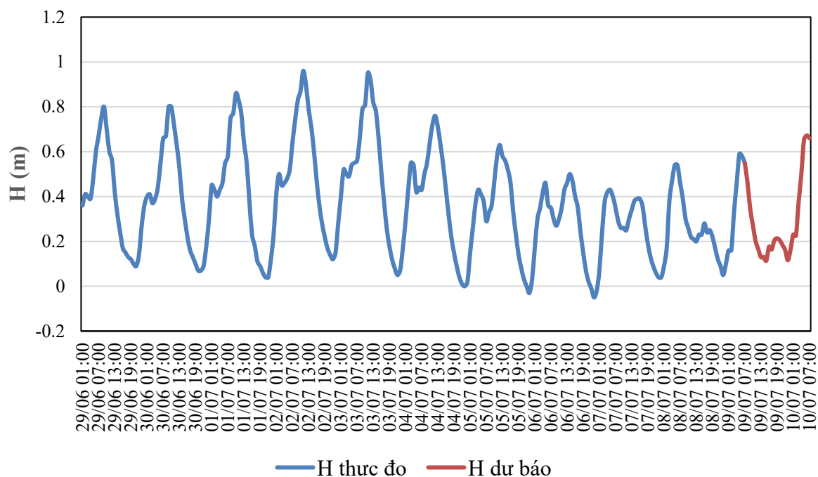
QUÁ TRÌNH MỨC NƯỚC THỰC ĐO VÀ DỰ BÁO TRẠM GIAO THỦY (Từ 01h/29/6 đến 07h/10/7/2026)
