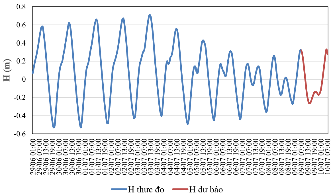
QUÁ TRÌNH MỨC NƯỚC THỰC ĐO VÀ DỰ BÁO TRẠM TAM KỲ (Từ 01h/29/6 đến 07h/10/7/2026)
