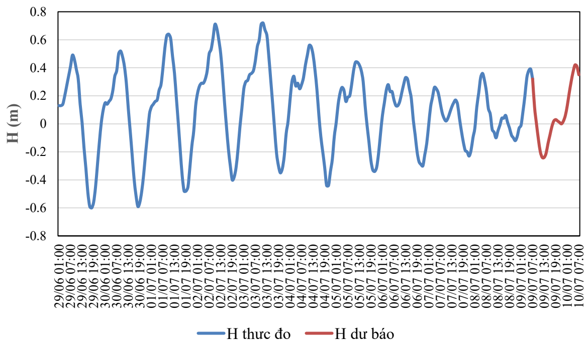
QUÁ TRÌNH MỨC NƯỚC THỰC ĐO VÀ DỰ BÁO TRẠM CÂU LÂU (Từ 01h/29/6 đến 07h/10/7/2026)
