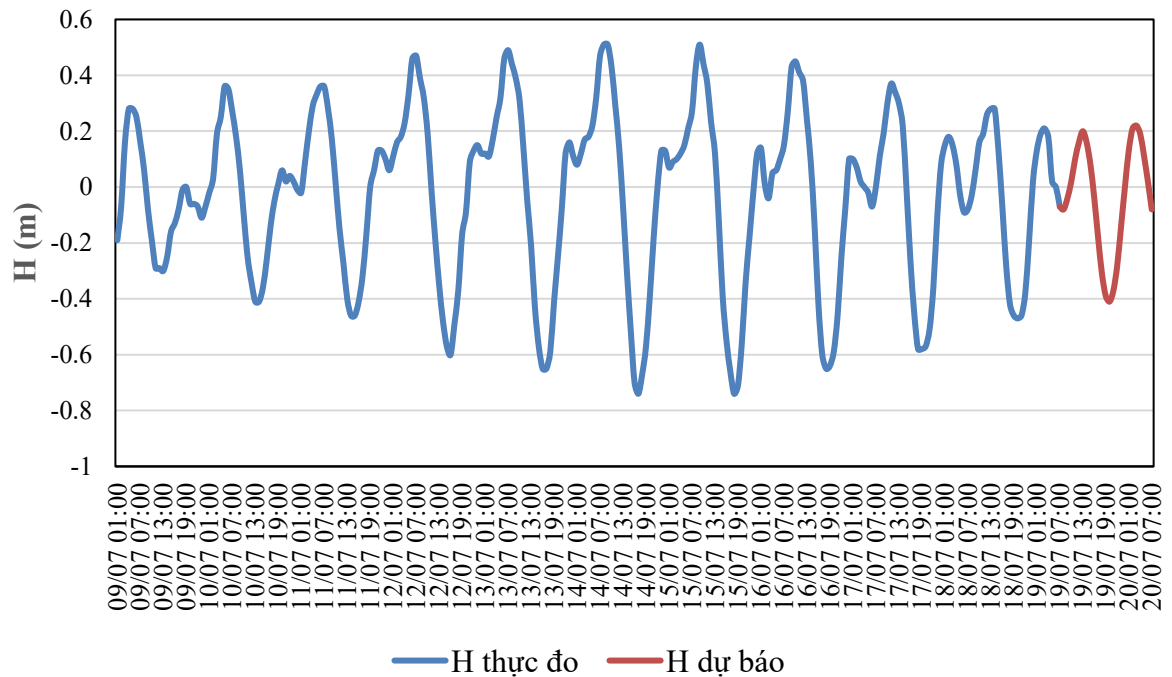
QUÁ TRÌNH MỨC NƯỚC THỰC ĐO VÀ DỰ BÁO TRẠM CẨM LỆ (Từ 01h/9/7 đến 07h/20/7/2026)
