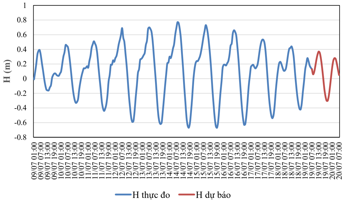
QUÁ TRÌNH MỨC NƯỚC THỰC ĐO VÀ DỰ BÁO TRẠM CÂU LÂU (Từ 01h/9/7 đến 07h/20/7/2026)
