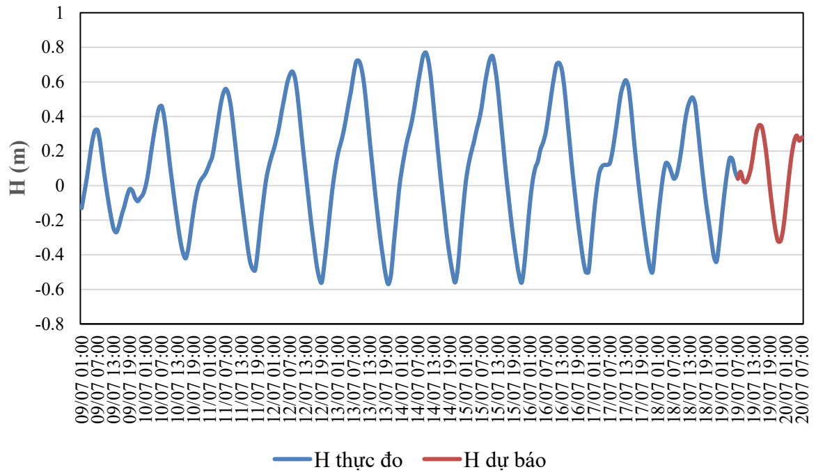
QUÁ TRÌNH MỨC NƯỚC THỰC ĐO VÀ DỰ BÁO TRẠM TAM KỲ (Từ 01h/9/7 đến 07h/20/7/2026)
