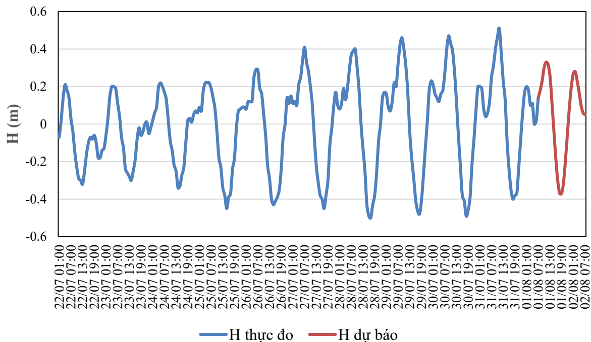
QUÁ TRÌNH MỰC NƯỚC THỰC ĐO VÀ DỰ BÁO TRẠM CẨM LỆ (Từ 01h/22/7 đến 07h/2/8/2026)
