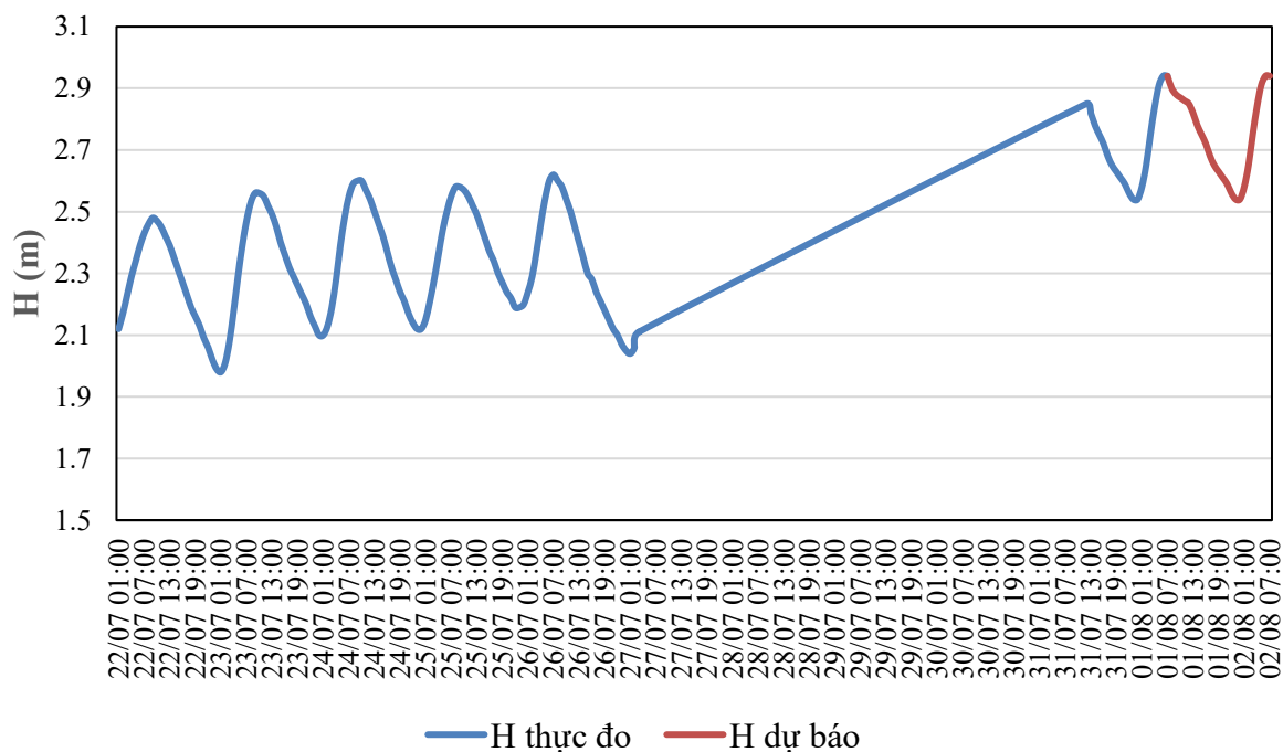
QUÁ TRÌNH MỰC NƯỚC THỰC ĐO VÀ DỰ BÁO TRẠM ÁI NGHĨA (Từ 01h/22/7 đến 07h/2/8/2026)
