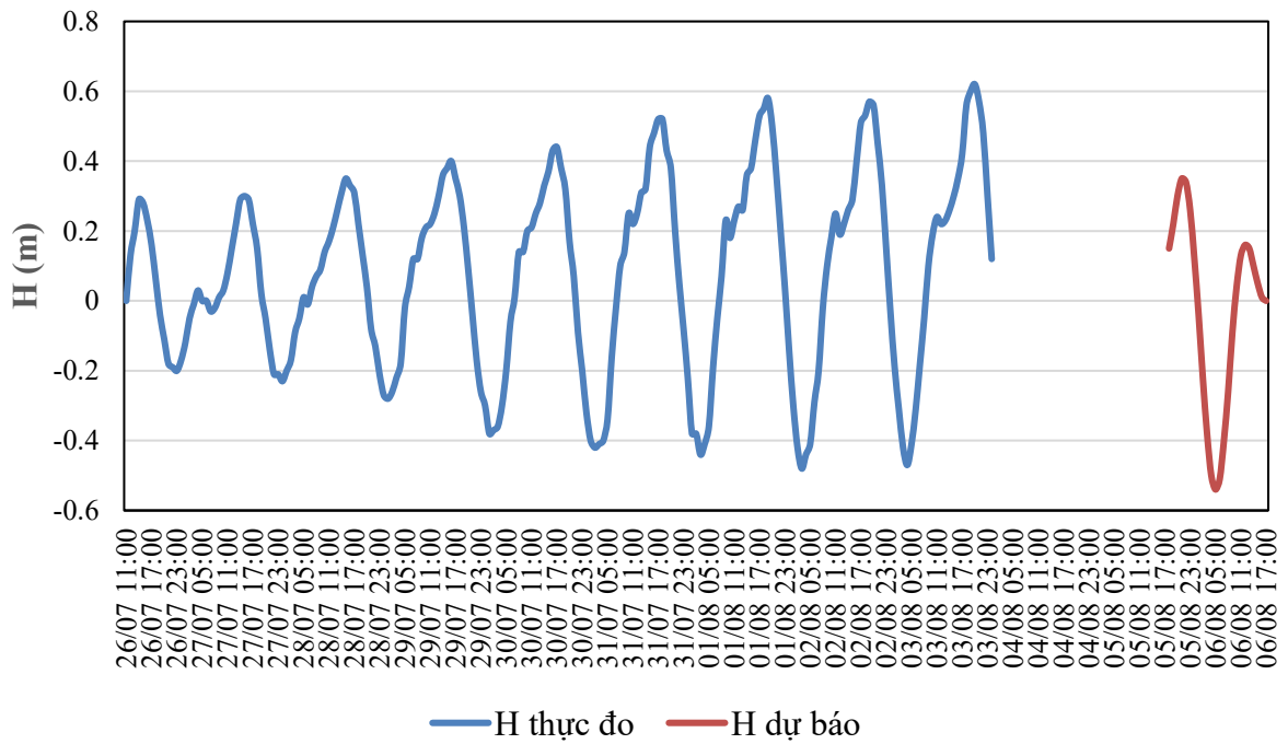
QUÁ TRÌNH MỨC NƯỚC THỰC ĐO VÀ DỰ BÁO TRẠM CÂU LÂU (Từ 01h/22/7 đến 07h/2/8/2026)
