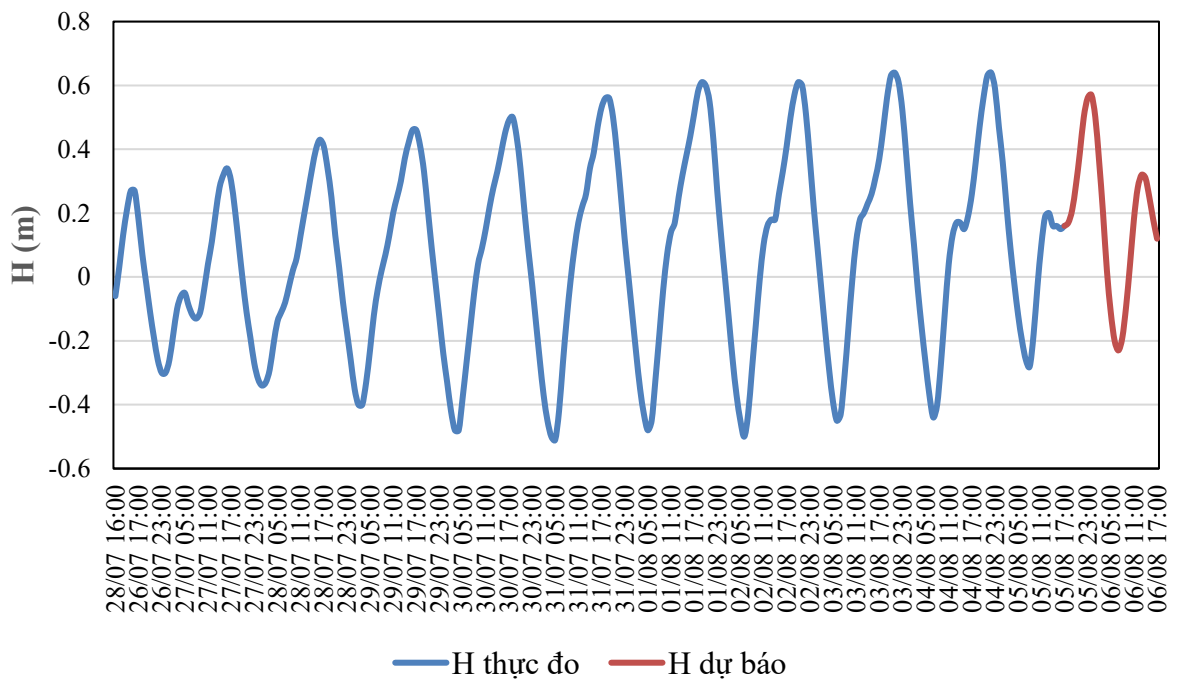
QUÁ TRÌNH MỨC NƯỚC THỰC ĐO VÀ DỰ BÁO TRẠM TAM KỲ (Từ 01h/22/7 đến 07h/2/8/2026)
