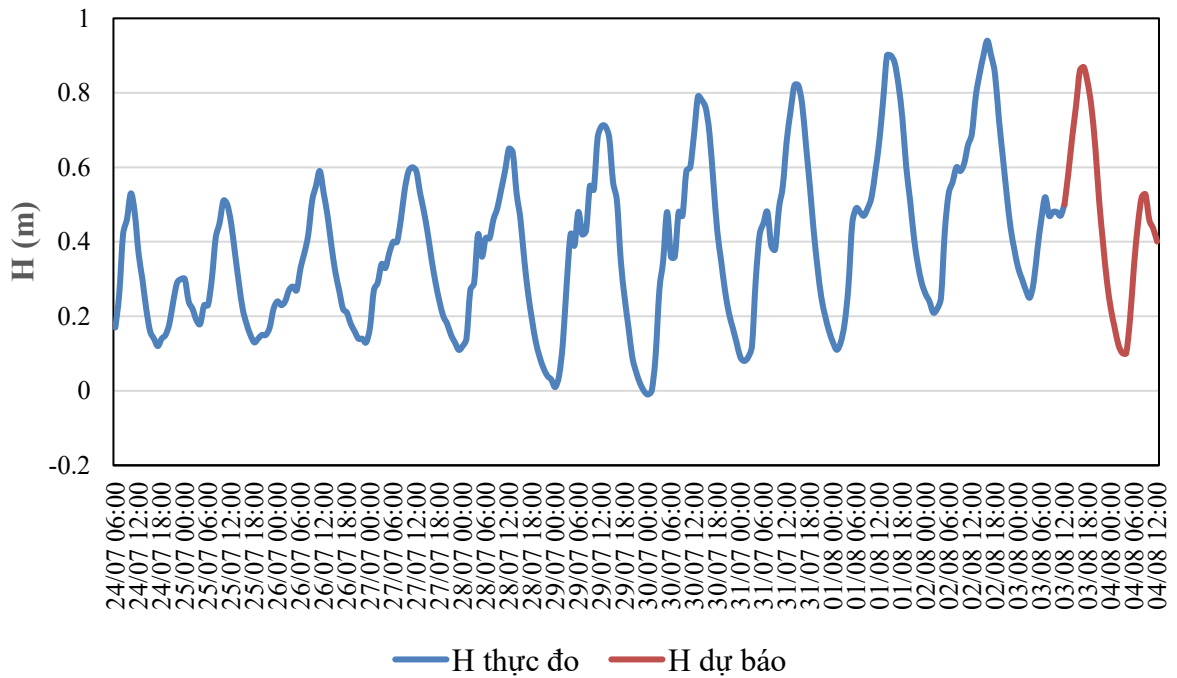
QUÁ TRÌNH MỨC NƯỚC THỰC ĐO VÀ DỰ BÁO TRẠM GIAO THỦY (Từ 01h/22/7 đến 07h/2/8/2026)
