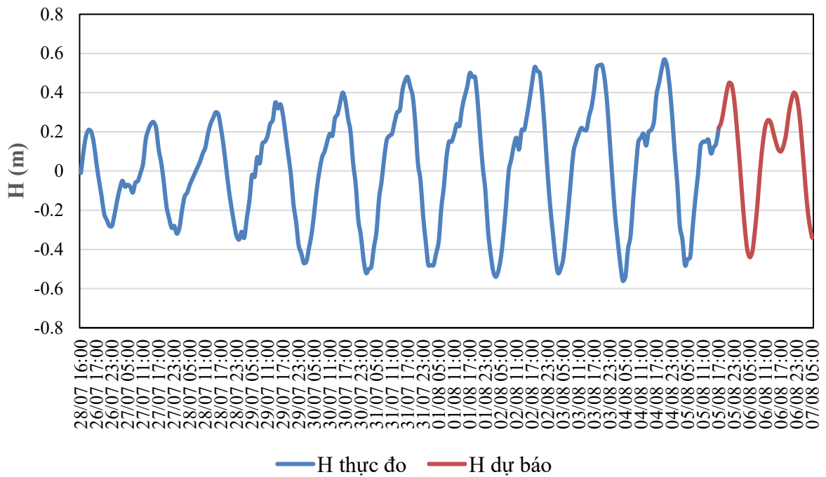
QUÁ TRÌNH MỨC NƯỚC THỰC ĐO VÀ DỰ BÁO TRẠM HỘI AN (Từ 01h/22/7 đến 07h/2/8/2026)
