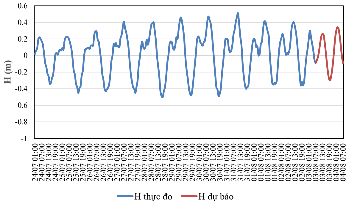
QUÁ TRÌNH MỨC NƯỚC THỰC ĐO VÀ DỰ BÁO TRẠM CẨM LỆ (Từ 01h/24/7 đến 07h/4/8/2026)
