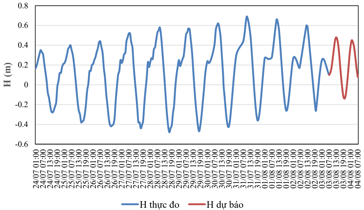
QUÁ TRÌNH MỨC NƯỚC THỰC ĐO VÀ DỰ BÁO TRẠM CÂU LÂU (Từ 01h/24/7 đến 07h/4/8/2026)
