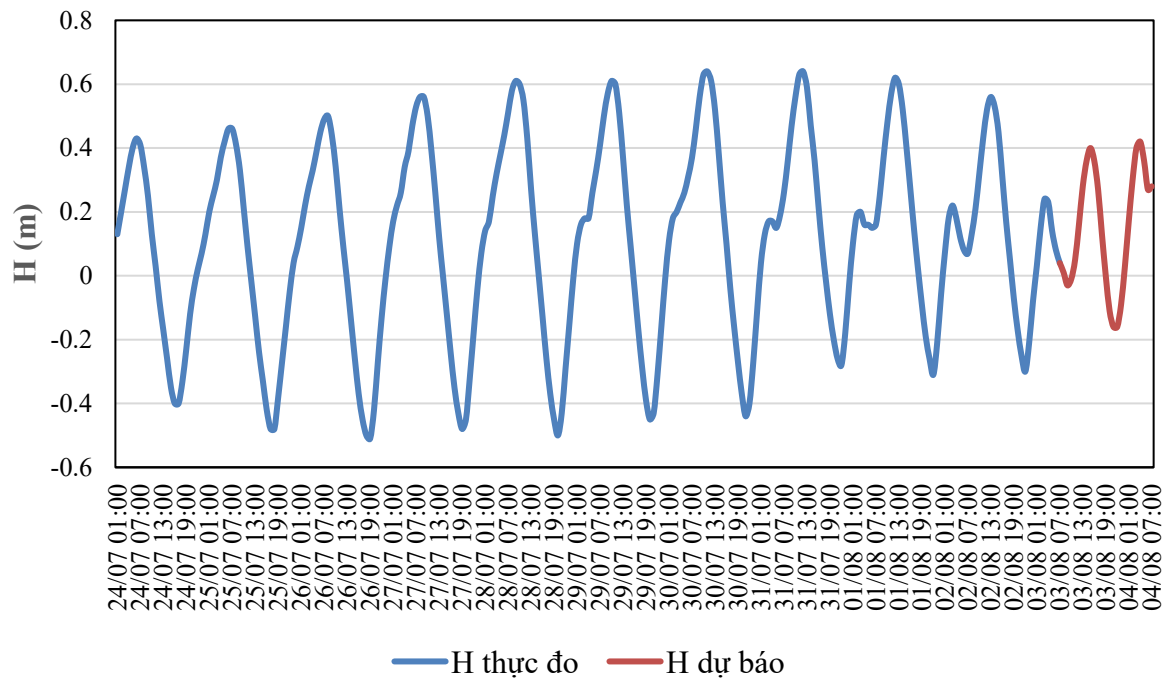
QUÁ TRÌNH MỨC NƯỚC THỰC ĐO VÀ DỰ BÁO TRẠM TAM KỲ (Từ 01h/24/7 đến 07h/4/8/2026)
