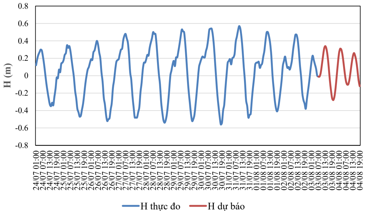
QUÁ TRÌNH MỨC NƯỚC THỰC ĐO VÀ DỰ BÁO TRẠM HỘI AN (Từ 01h/24/7 đến 07h/4/8/2026)
