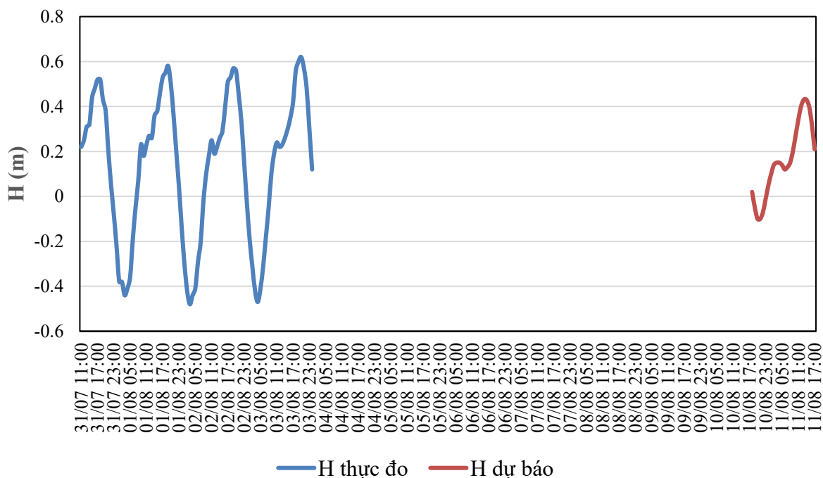
QUÁ TRÌNH MỨC NƯỚC THỰC ĐO VÀ DỰ BÁO TRẠM CÂU LÂU (Từ 01h/27/7 đến 07h/7/8/2026)
