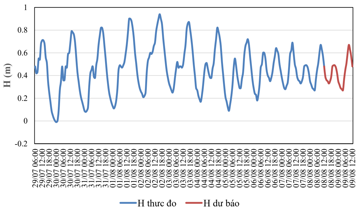
QUÁ TRÌNH MỨC NƯỚC THỰC ĐO VÀ DỰ BÁO TRẠM GIAO THỦY (Từ 01h/27/7 đến 07h/7/8/2026)
