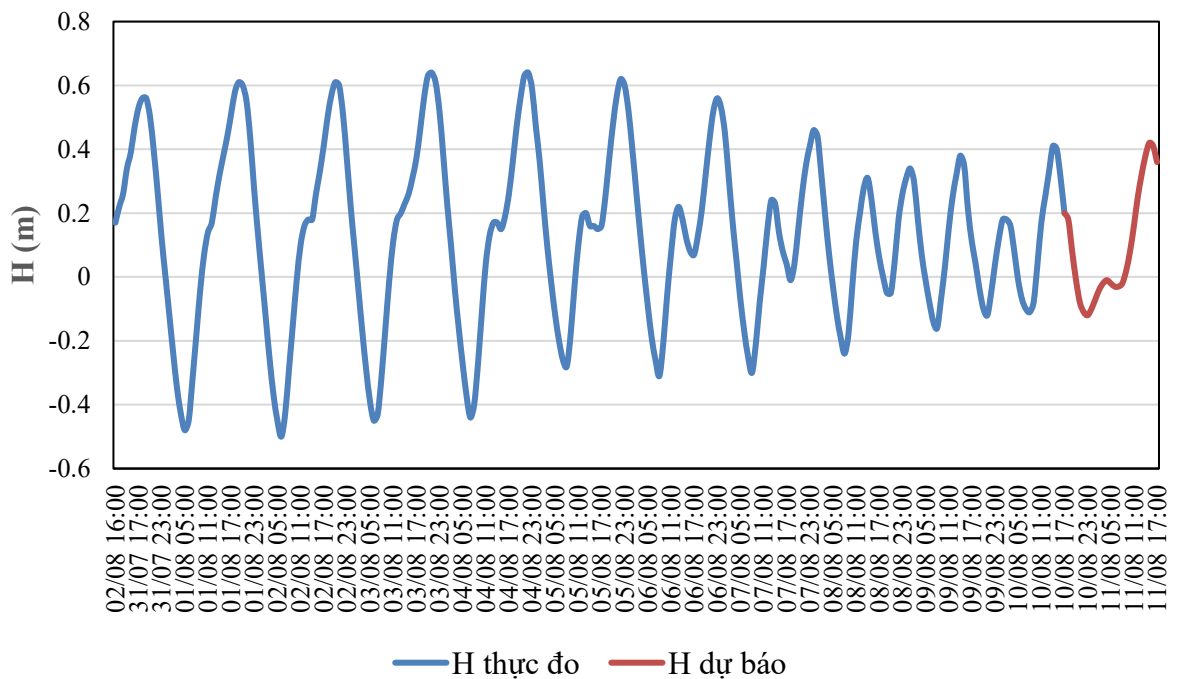
QUÁ TRÌNH MỨC NƯỚC THỰC ĐO VÀ DỰ BÁO TRẠM TAM KỲ (Từ 01h/27/7 đến 07h/7/8/2026)
