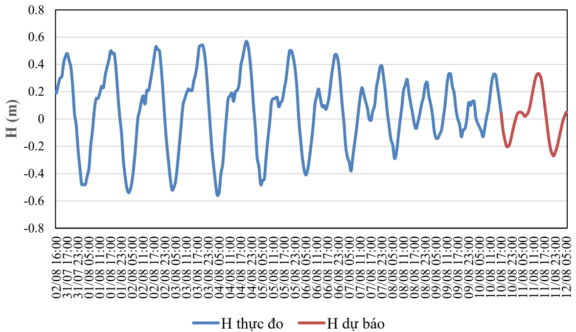
QUÁ TRÌNH MỨC NƯỚC THỰC ĐO VÀ DỰ BÁO TRẠM HỘI AN (Từ 01h/27/7 đến 07h/7/8/2026)
