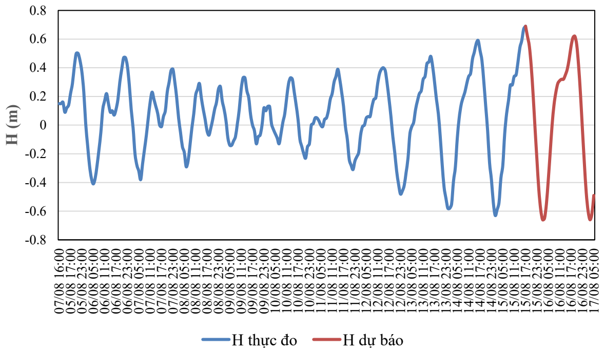
QUÁ TRÌNH MỨC NƯỚC THỰC ĐO VÀ DỰ BÁO TRẠM HỘI AN (Từ 01h/1/8 đến 07h/12/8/2026)
