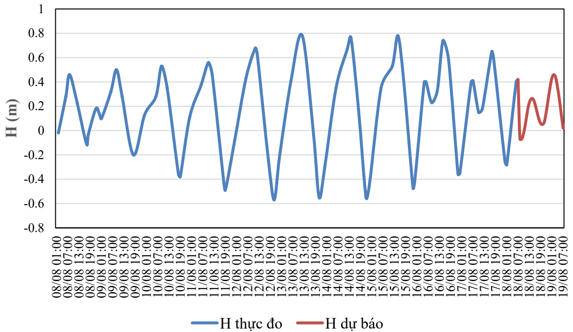
QUÁ TRÌNH MỨC NƯỚC THỰC ĐO VÀ DỰ BÁO TRẠM CÂU LÂU (Từ 01h/8/8 đến 07h/19/8/2026)
