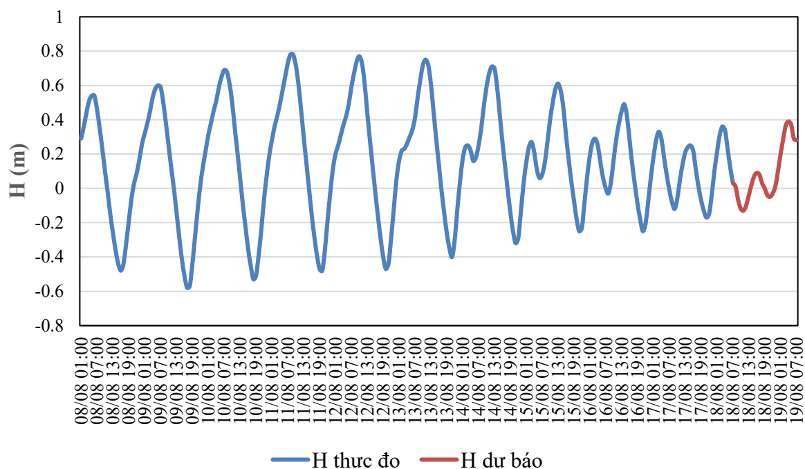
QUÁ TRÌNH MỨC NƯỚC THỰC ĐO VÀ DỰ BÁO TRẠM TAM KỲ (Từ 01h/8/8 đến 07h/19/8/2026)
