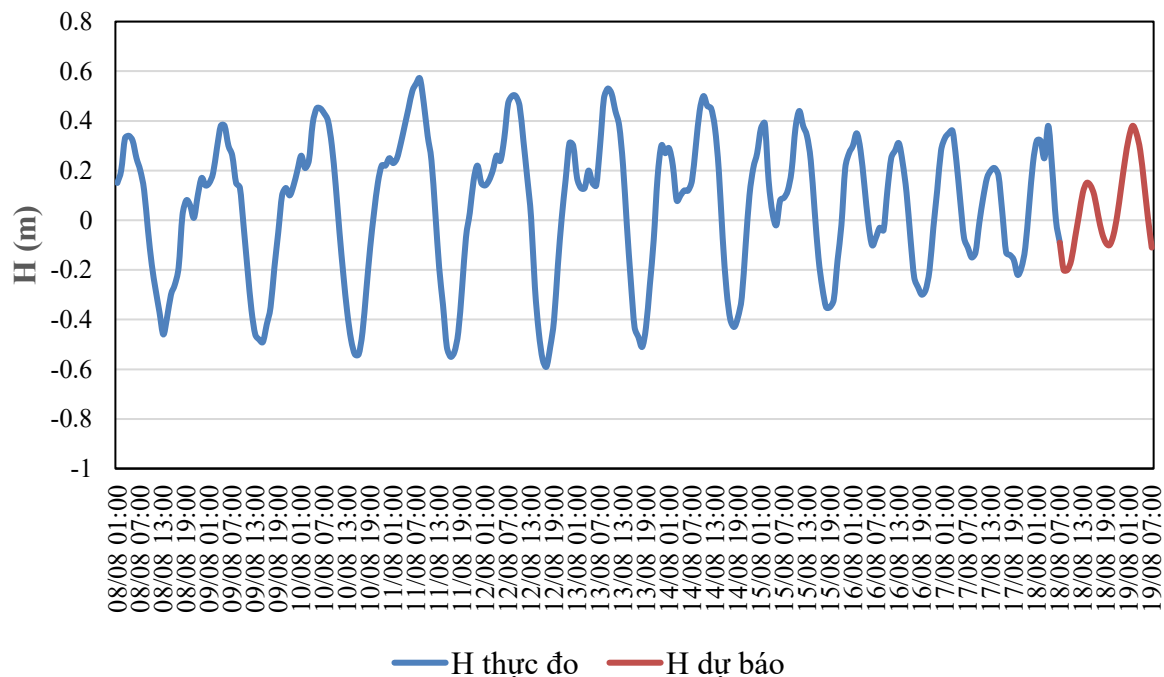
QUÁ TRÌNH MỨC NƯỚC THỰC ĐO VÀ DỰ BÁO TRẠM CẨM LỆ (Từ 01h/8/8 đến 07h/19/8/2026)
