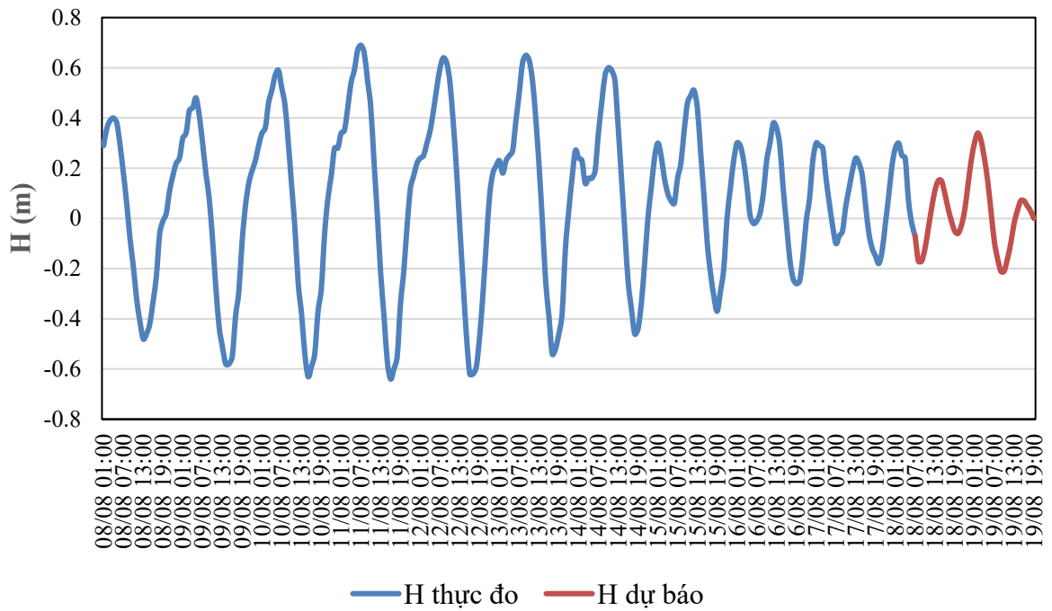
QUÁ TRÌNH MỨC NƯỚC THỰC ĐO VÀ DỰ BÁO TRẠM HỘI AN (Từ 01h/8/8 đến 07h/19/8/2026)
