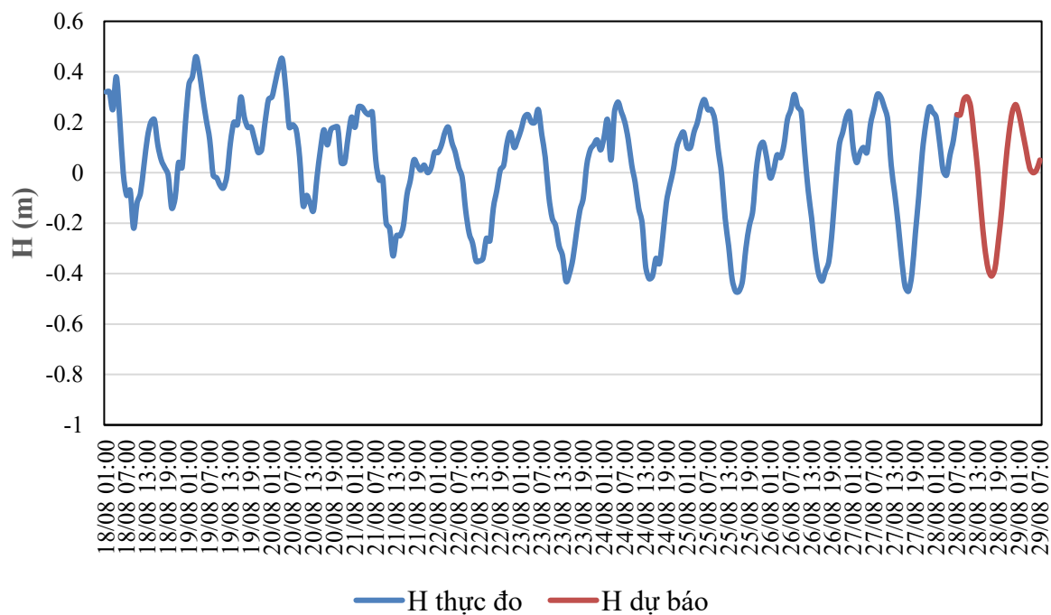
QUÁ TRÌNH MỨC NƯỚC THỰC ĐO VÀ DỰ BÁO TRẠM CẨM LỆ (Từ 01h/18/8 đến 07h/29/8/2026)
