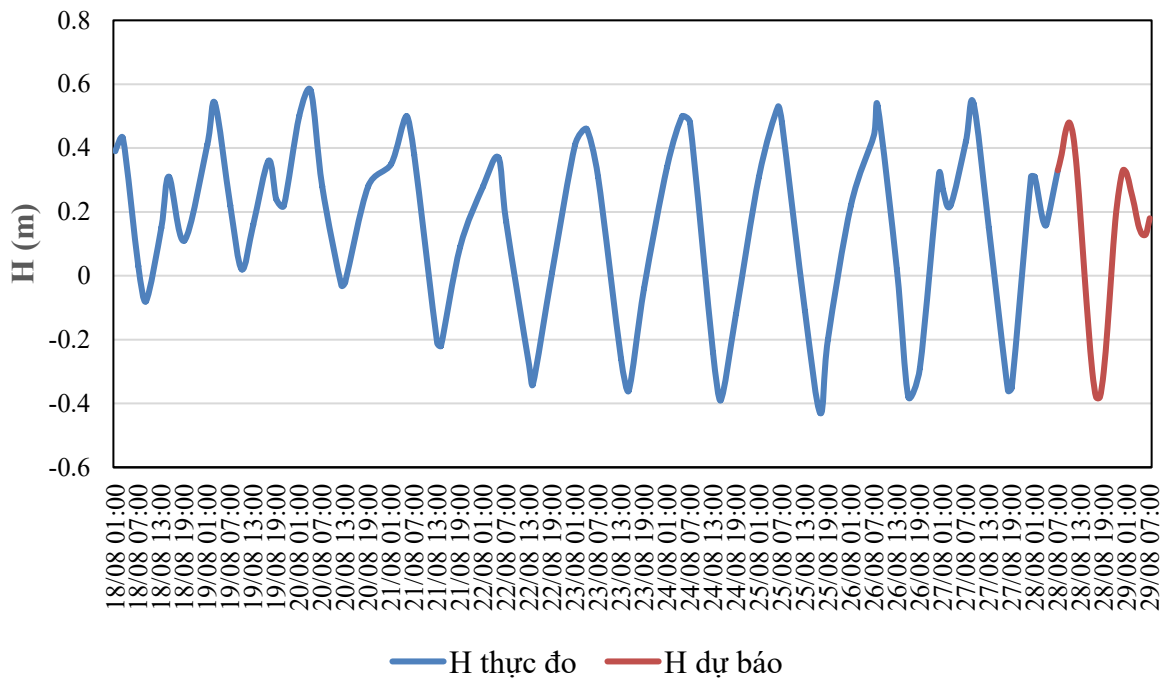
QUÁ TRÌNH MỨC NƯỚC THỰC ĐO VÀ DỰ BÁO TRẠM CÂU LÂU (Từ 01h/18/8 đến 07h/29/8/2026)
