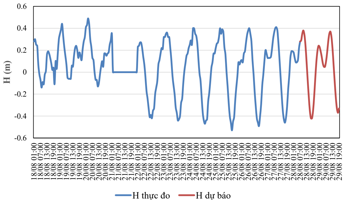
QUÁ TRÌNH MỨC NƯỚC THỰC ĐO VÀ DỰ BÁO TRẠM HỘI AN (Từ 01h/18/8 đến 07h/29/8/2026)
