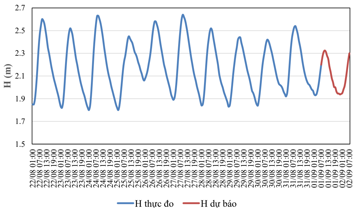
QUÁ TRÌNH MỰC NƯỚC THỰC ĐO VÀ DỰ BÁO TRẠM ÁI NGHĨA (Từ 01h/22/8 đến 07h/2/9/2026)
