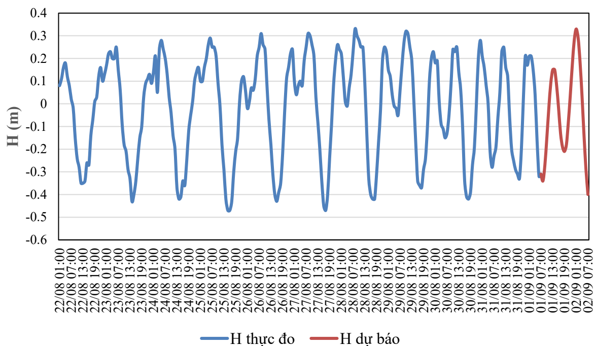
QUÁ TRÌNH MỰC NƯỚC THỰC ĐO VÀ DỰ BÁO TRẠM CẨM LỆ (Từ 01h/22/8 đến 07h/2/9/2026)
