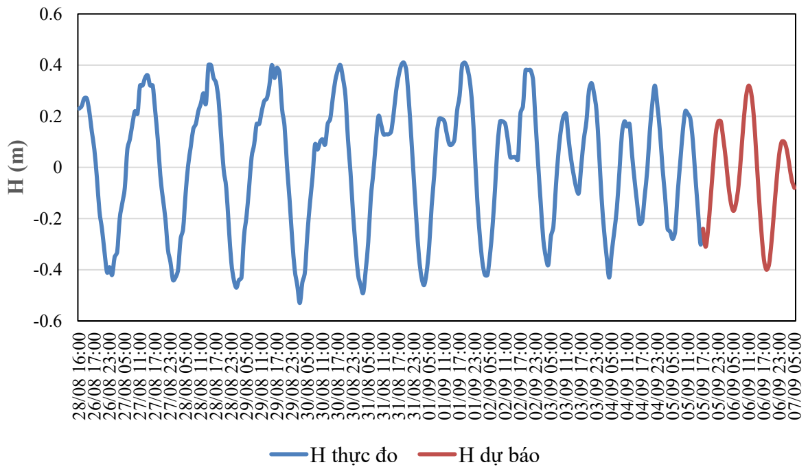
QUÁ TRÌNH MỨC NƯỚC THỰC ĐO VÀ DỰ BÁO TRẠM HỘI AN (Từ 01h/22/8 đến 07h/2/9/2026)
