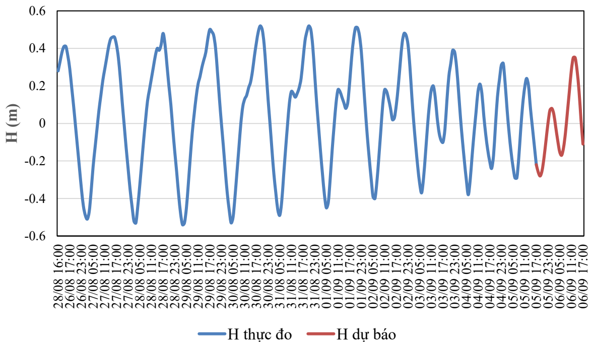
QUÁ TRÌNH MỨC NƯỚC THỰC ĐO VÀ DỰ BÁO TRẠM TAM KỲ (Từ 01h/22/8 đến 07h/2/9/2026)
