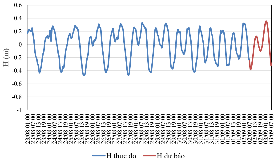
QUÁ TRÌNH MỨC NƯỚC THỰC ĐO VÀ DỰ BÁO TRẠM CẨM LỆ (Từ 01h/23/8 đến 07h/3/9/2026)
