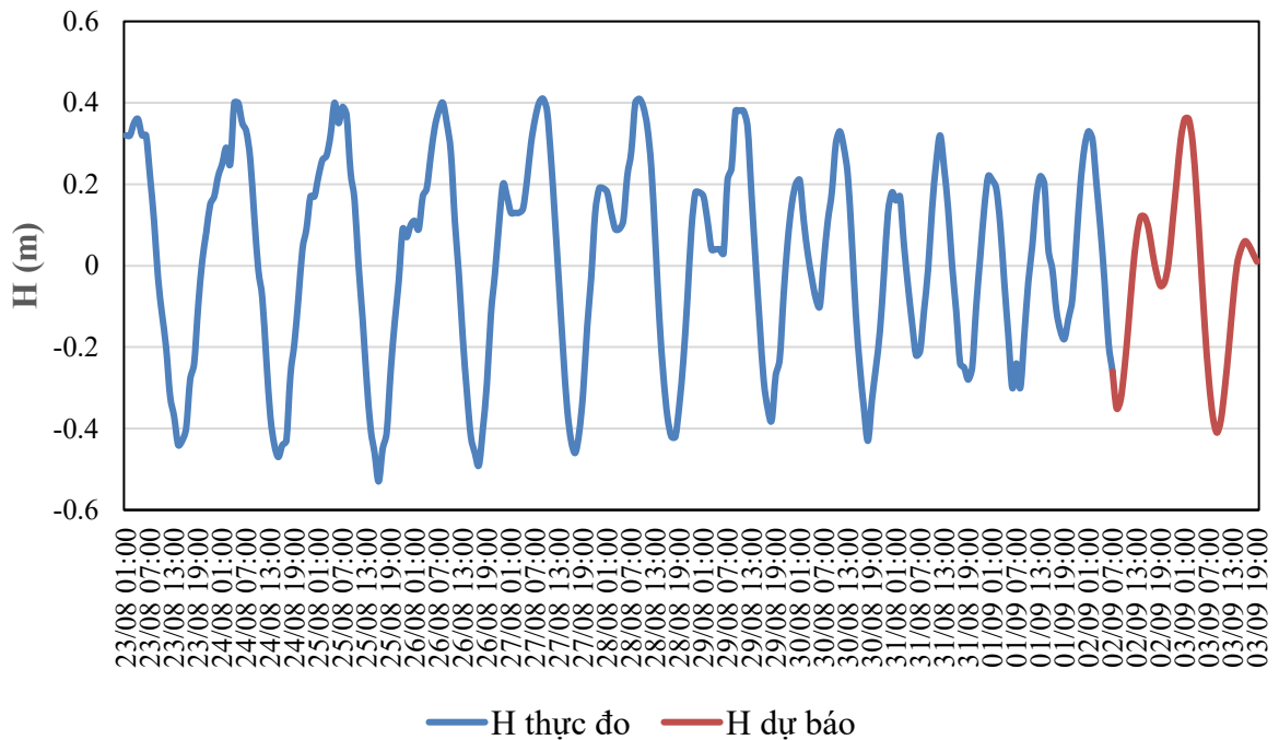
QUÁ TRÌNH MỨC NƯỚC THỰC ĐO VÀ DỰ BÁO TRẠM HỘI AN (Từ 01h/23/8 đến 07h/3/9/2026)
