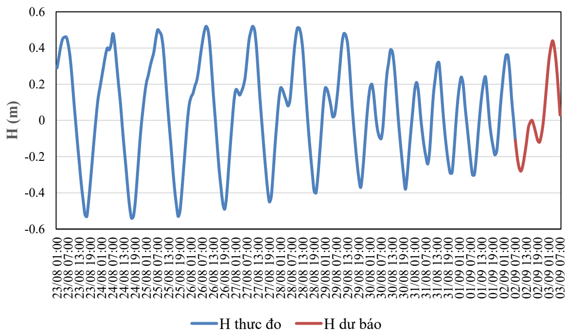
QUÁ TRÌNH MỨC NƯỚC THỰC ĐO VÀ DỰ BÁO TRẠM TAM KỲ (Từ 01h/23/8 đến 07h/3/9/2026)
