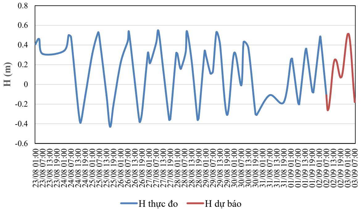
QUÁ TRÌNH MỨC NƯỚC THỰC ĐO VÀ DỰ BÁO TRẠM CÂU LÂU (Từ 01h/23/8 đến 07h/3/9/2026)
