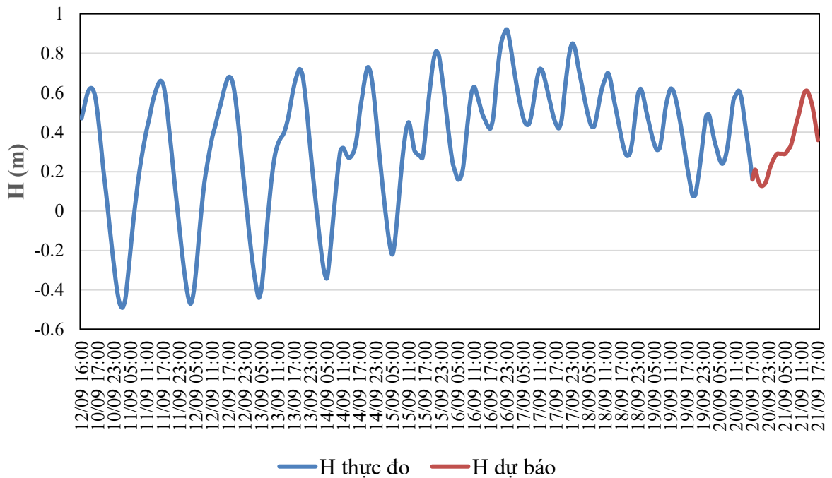
QUÁ TRÌNH MỨC NƯỚC THỰC ĐO VÀ DỰ BÁO TRẠM TAM KỲ (Từ 01h/6/9 đến 07h/17/9/2026)
