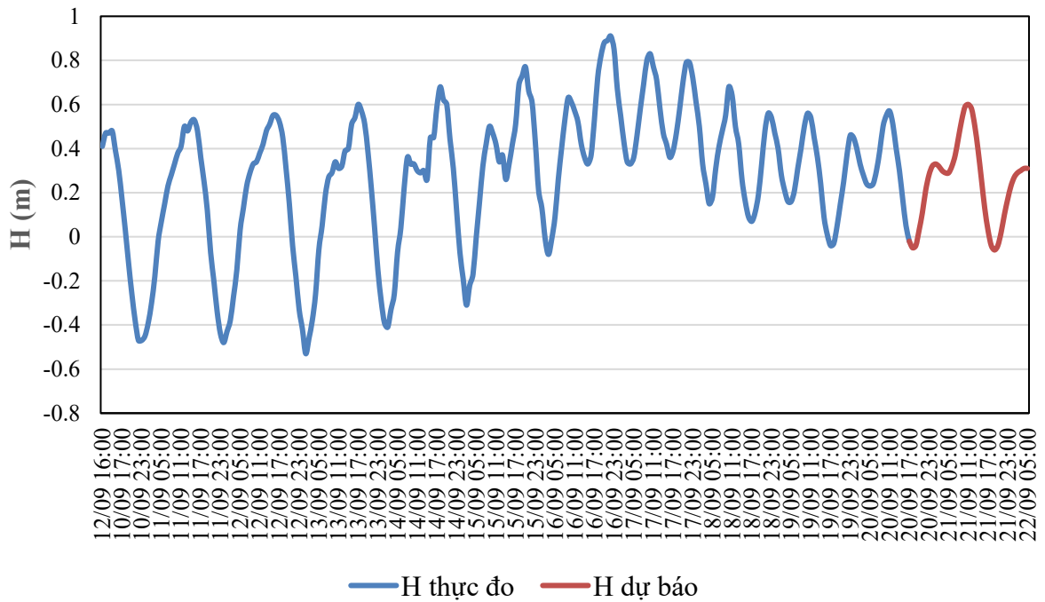
QUÁ TRÌNH MỨC NƯỚC THỰC ĐO VÀ DỰ BÁO TRẠM HỘI AN (Từ 01h/6/9 đến 07h/17/9/2026)
