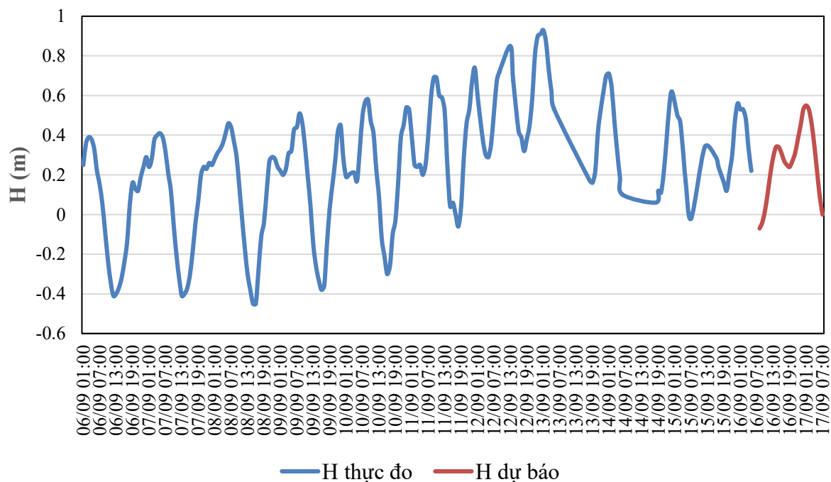
QUÁ TRÌNH MỰC NƯỚC THỰC ĐO VÀ DỰ BÁO TRẠM CẨM LỆ (Từ 01h/6/9 đến 07h/17/9/2026)
