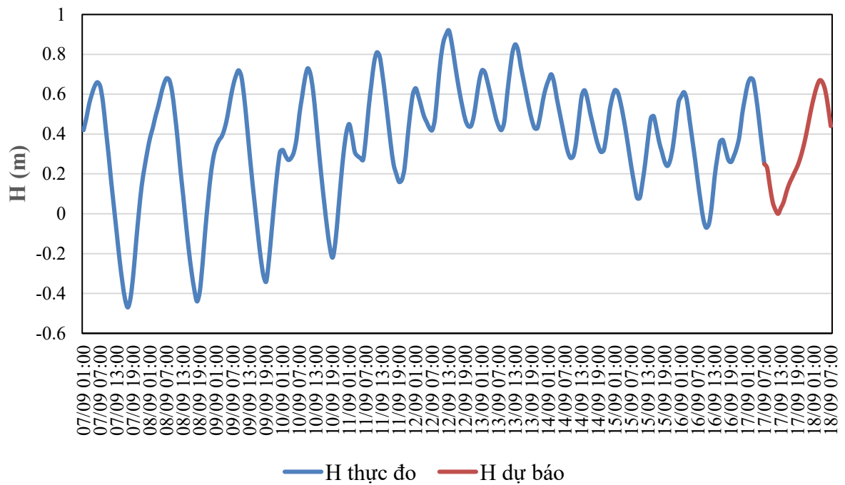
QUÁ TRÌNH MỨC NƯỚC THỰC ĐO VÀ DỰ BÁO TRẠM TAM KỲ (Từ 01h/7/9 đến 07h/18/9/2026)
