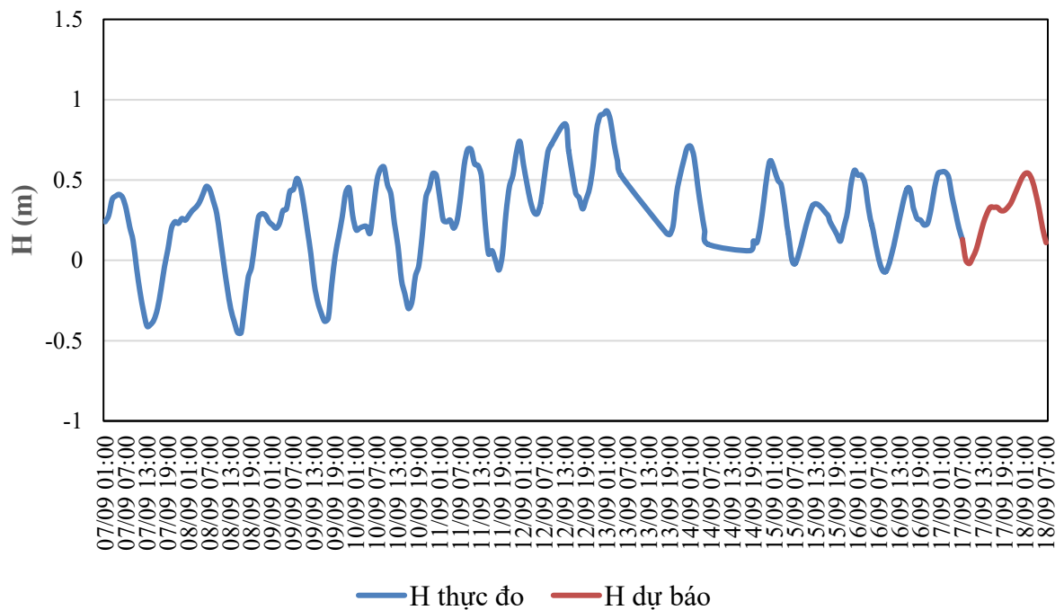
QUÁ TRÌNH MỨC NƯỚC THỰC ĐO VÀ DỰ BÁO TRẠM CẨM LỆ (Từ 01h/7/9 đến 07h/18/9/2026)
