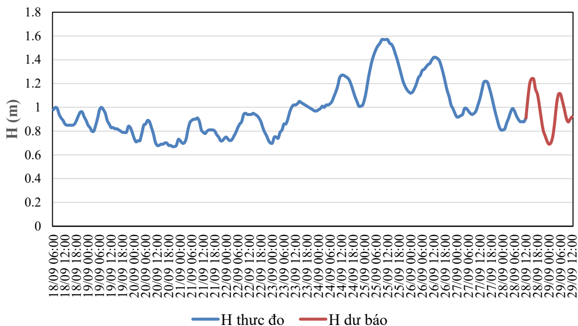
QUÁ TRÌNH MỨC NƯỚC THỰC ĐO VÀ DỰ BÁO TRẠM GIAO THỦY (Từ 01h/16/9 đến 07h/27/9/2026)
