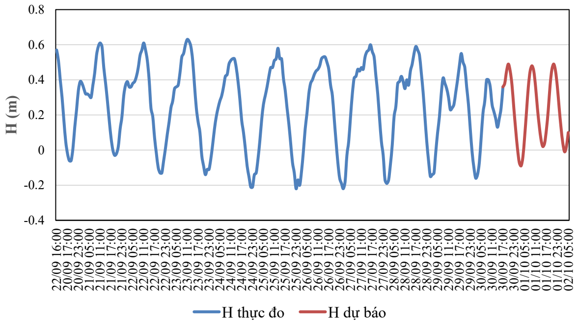
QUÁ TRÌNH MỨC NƯỚC THỰC ĐO VÀ DỰ BÁO TRẠM HỘI AN (Từ 01h/16/9 đến 07h/27/9/2026)
