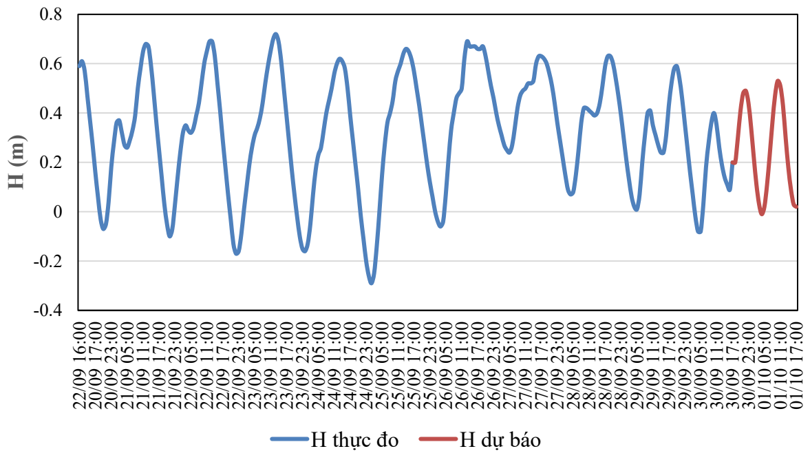
QUÁ TRÌNH MỨC NƯỚC THỰC ĐO VÀ DỰ BÁO TRẠM TAM KỲ (Từ 01h/16/9 đến 07h/27/9/2026)
