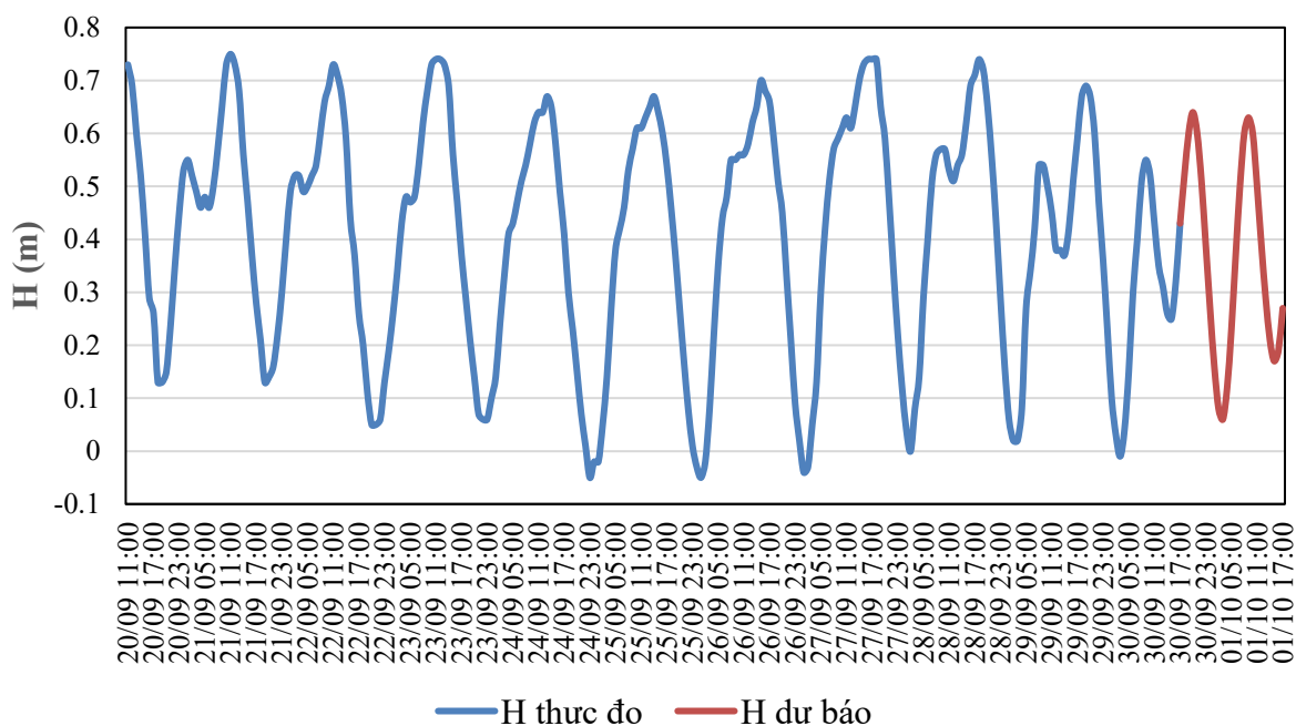
QUÁ TRÌNH MỨC NƯỚC THỰC ĐO VÀ DỰ BÁO TRẠM CÂU LÂU (Từ 01h/16/9 đến 07h/27/9/2026)
