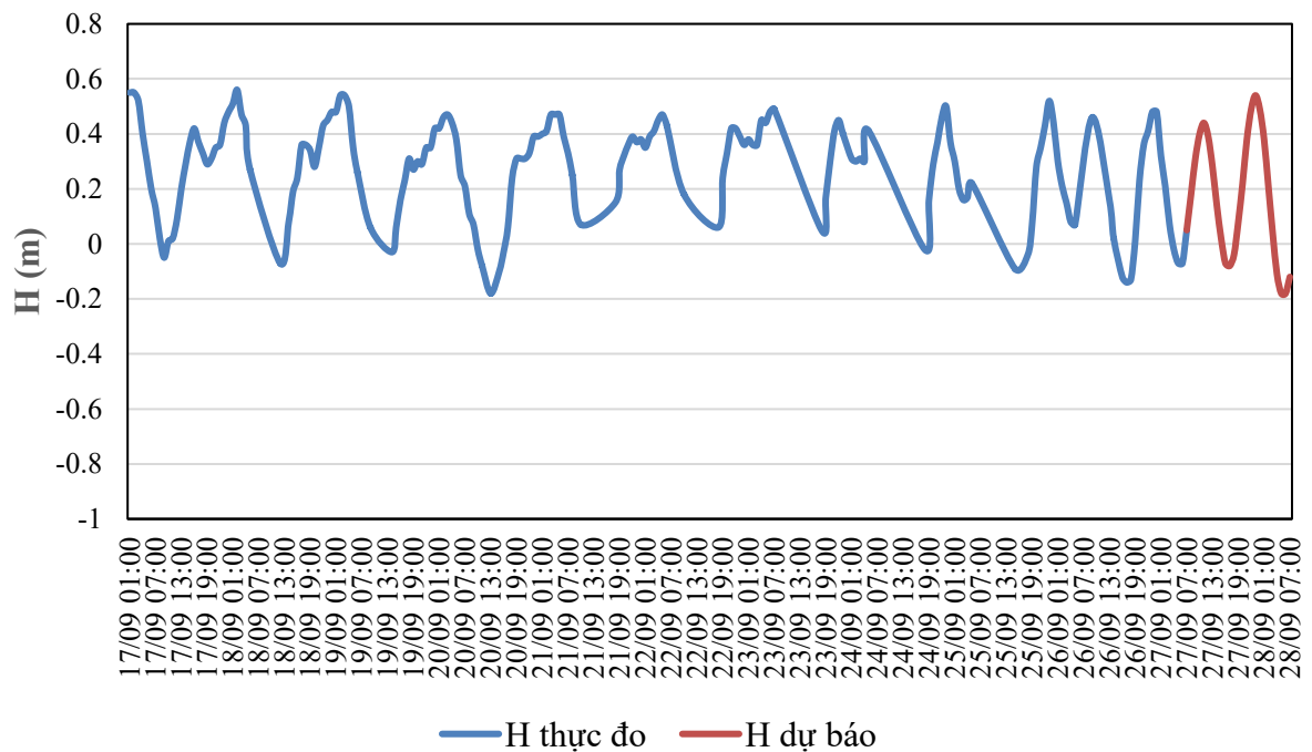
QUÁ TRÌNH MỨC NƯỚC THỰC ĐO VÀ DỰ BÁO TRẠM CẨM LỆ (Từ 01h/17/9 đến 07h/28/9/2026)
