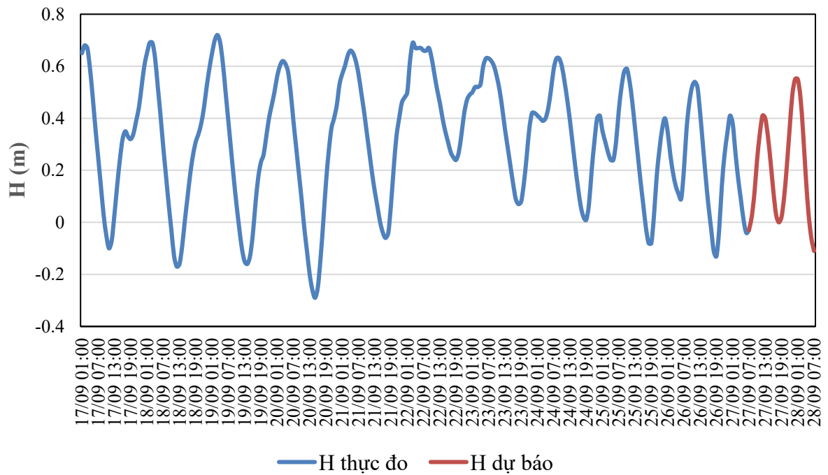
QUÁ TRÌNH MỨC NƯỚC THỰC ĐO VÀ DỰ BÁO TRẠM TAM KỲ (Từ 01h/17/9 đến 07h/28/9/2026)
