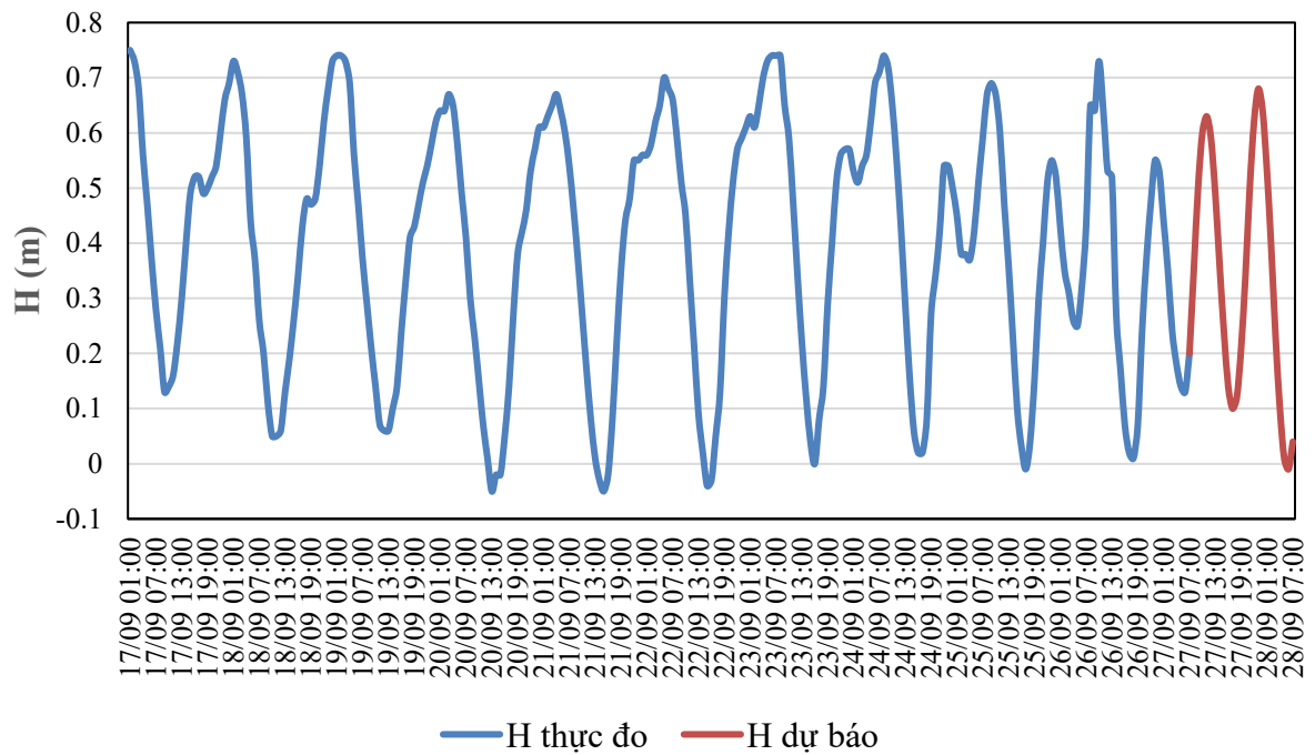
QUÁ TRÌNH MỨC NƯỚC THỰC ĐO VÀ DỰ BÁO TRẠM CÂU LÂU (Từ 01h/17/9 đến 07h/28/9/2026)
