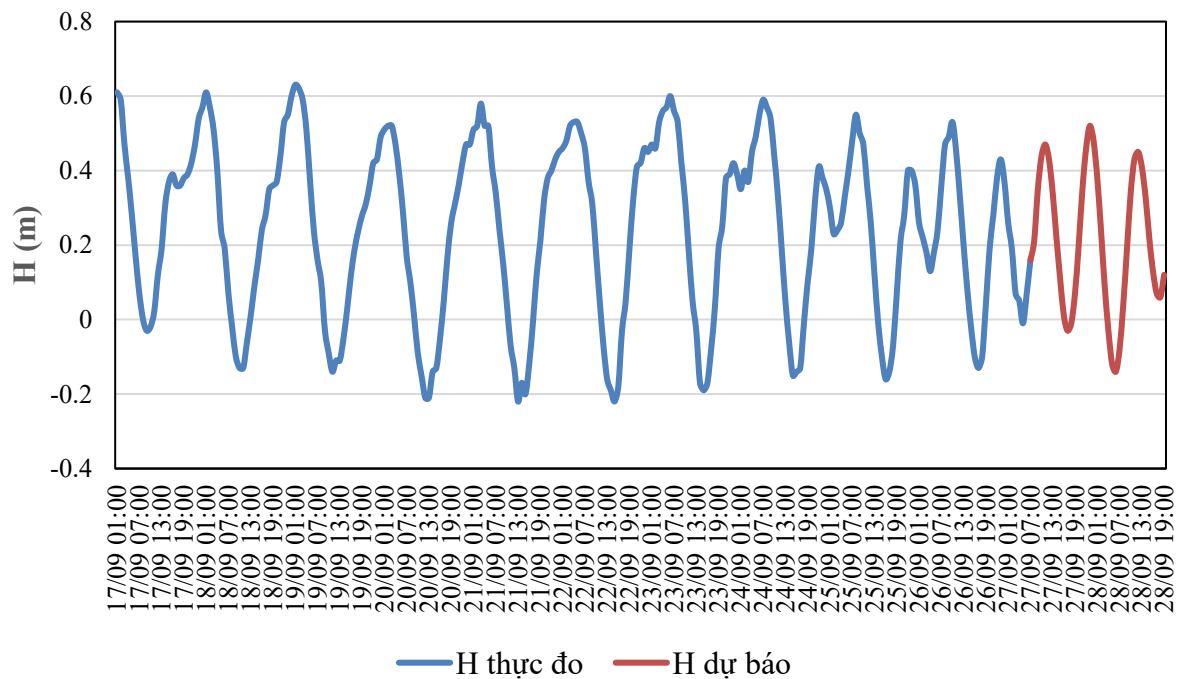
QUÁ TRÌNH MỨC NƯỚC THỰC ĐO VÀ DỰ BÁO TRẠM HỘI AN (Từ 01h/17/9 đến 07h/28/9/2026)
