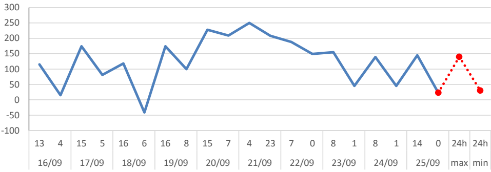
Quá trình mực nước thực đo và dự báo trạm Chợ Tràng
