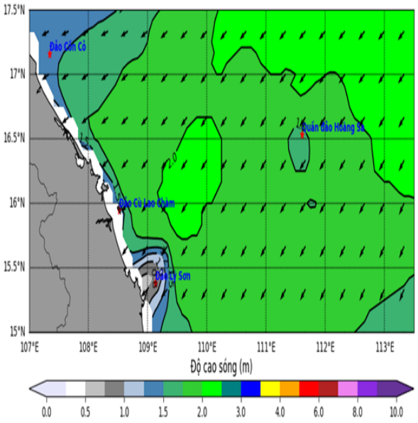
Hình 1: Bản đồ dự báo gió mạnh 24 giờ tới Hình 2: Bản đồ dự báo sóng lớn 24 giờ tới
