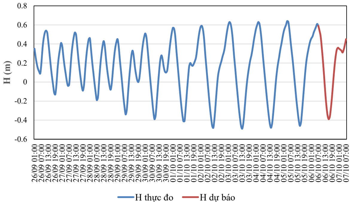
QUÁ TRÌNH MỨC NƯỚC THỰC ĐO VÀ DỰ BÁO TRẠM TAM KỲ (Từ 01h/26/9 đến 07h/7/10/2026)
