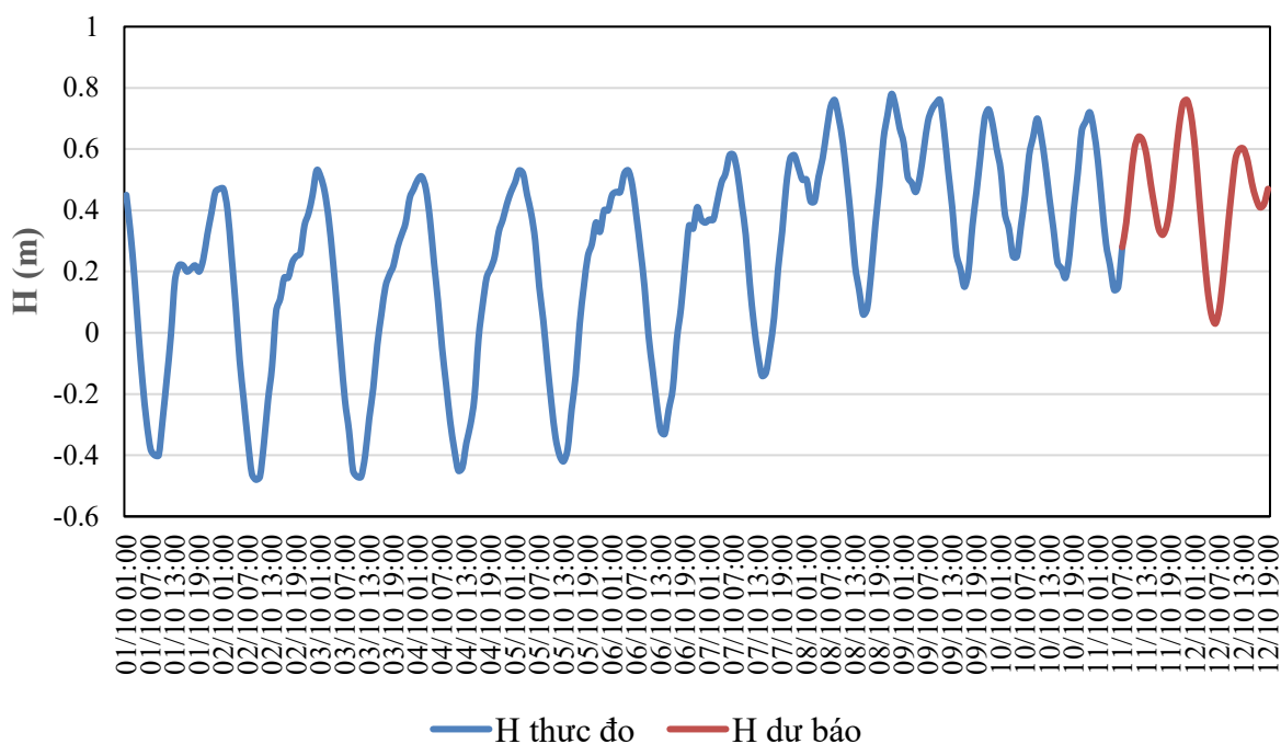
QUÁ TRÌNH MỨC NƯỚC THỰC ĐO VÀ DỰ BÁO TRẠM HỘI AN (Từ 01h/1/10 đến 07h/12/10/2026)
