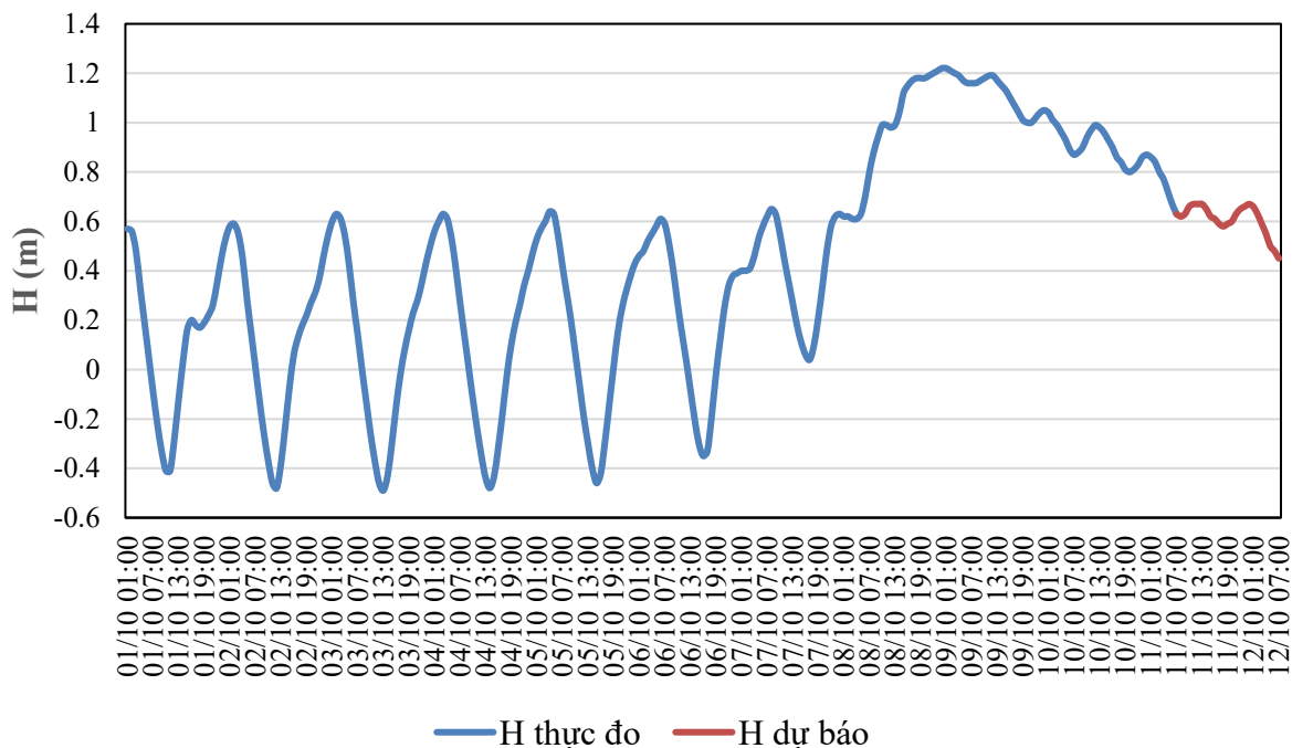
QUÁ TRÌNH MỨC NƯỚC THỰC ĐO VÀ DỰ BÁO TRẠM TAM KỲ (Từ 01h/1/10 đến 07h/12/10/2026)
