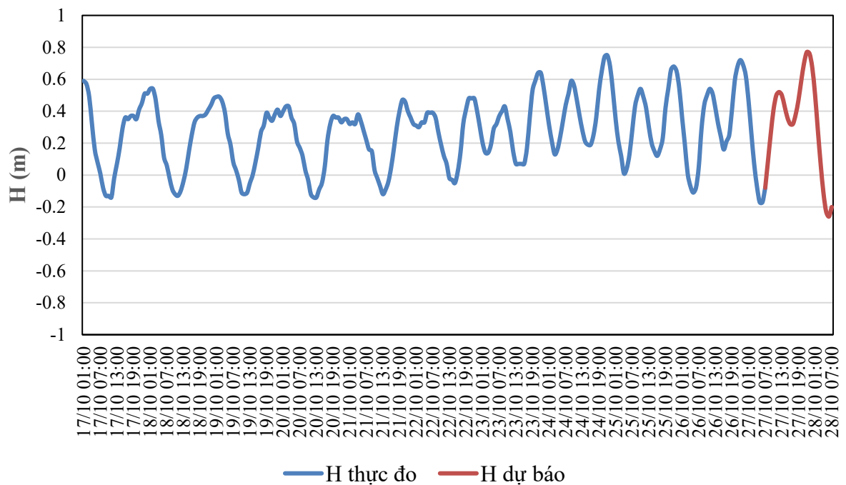
QUÁ TRÌNH MỨC NƯỚC THỰC ĐO VÀ DỰ BÁO TRẠM CẨM LỆ (Từ 01h/17/10 đến 07h/28/10/2026)
