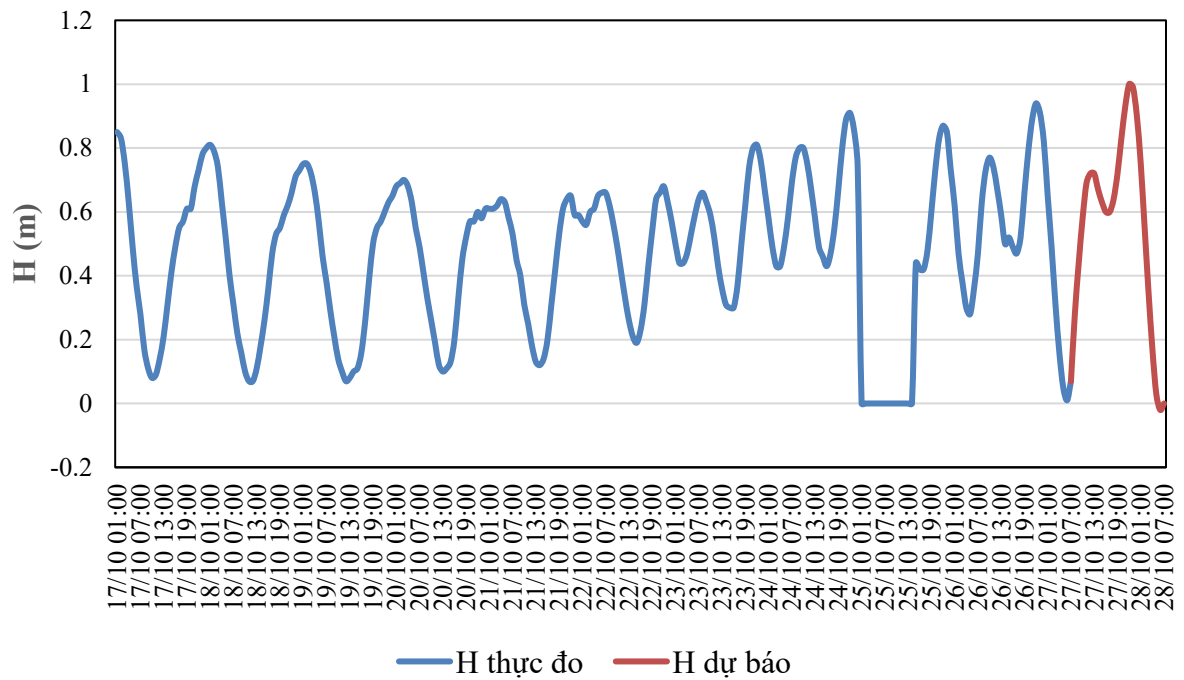
QUÁ TRÌNH MỨC NƯỚC THỰC ĐO VÀ DỰ BÁO TRẠM CÂU LÂU (Từ 01h/17/10 đến 07h/28/10/2026)
