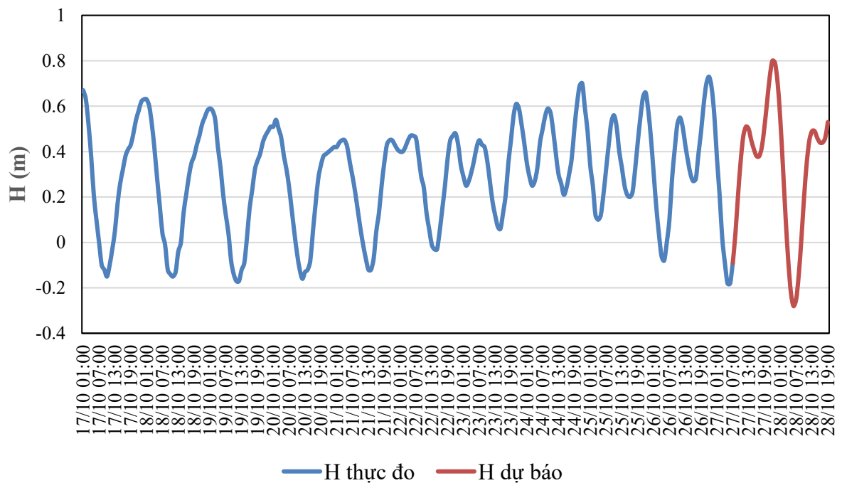
QUÁ TRÌNH MỨC NƯỚC THỰC ĐO VÀ DỰ BÁO TRẠM HỘI AN (Từ 01h/17/10 đến 07h/28/10/2026)
