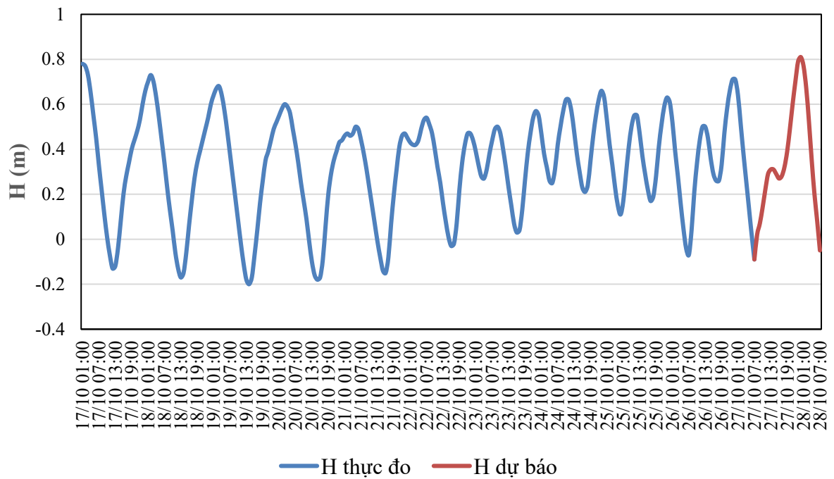
QUÁ TRÌNH MỨC NƯỚC THỰC ĐO VÀ DỰ BÁO TRẠM TAM KỲ (Từ 01h/17/10 đến 07h/28/10/2026)
